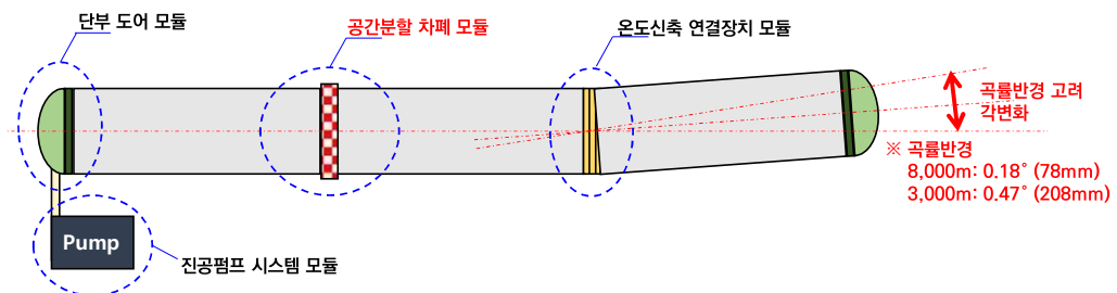
<아진공 튜브 Mock-Up의 기본 형상 및 장치 구성 예시>
