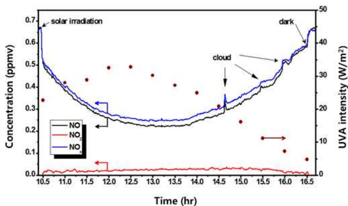
그림 13. 광촉매 대기정화 성능평가 실험
