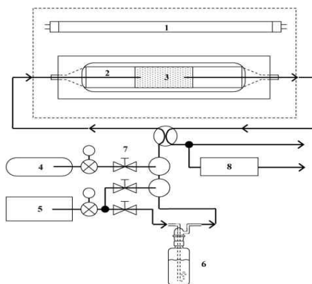
그림 72. ISO 22197-1 시험방법
