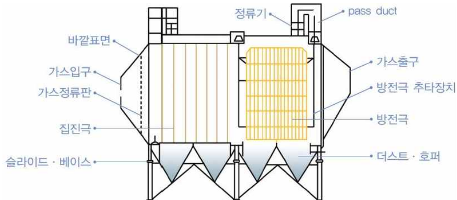
그림 66. 전기집진기 개요도(예)
