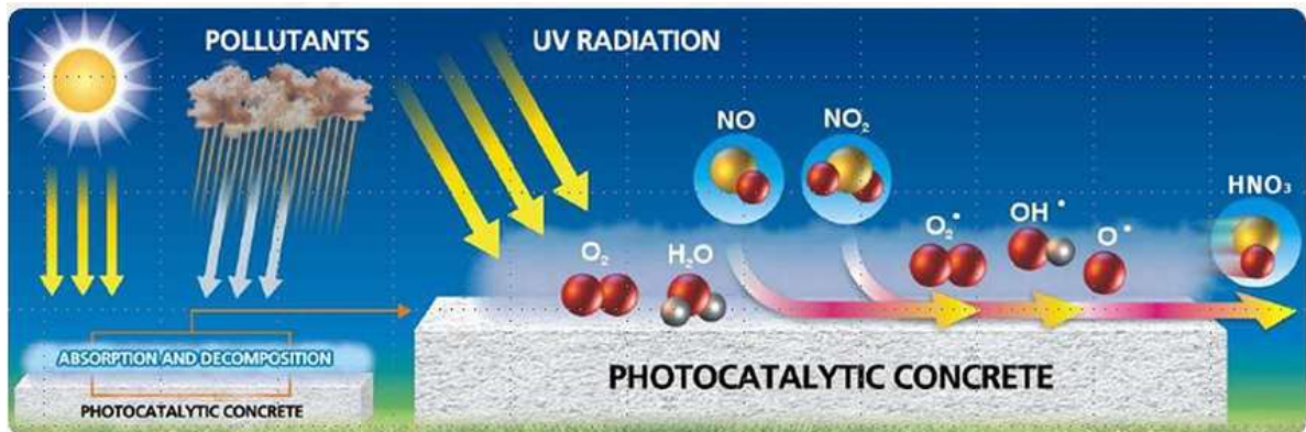
그림 5. 광촉매 콘크리트의 대기정화 개념
