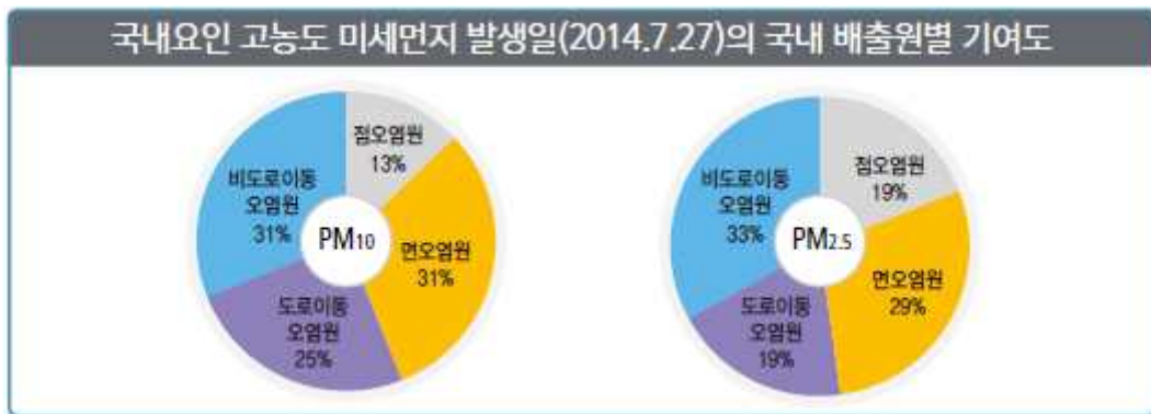
그림 17. 미세먼지 발생 배출원 분포 (2014년)
