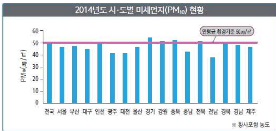
그림 16. 시도별 미세먼지( PM_{10} ) 현황(2014년) (출처: 미세먼지의 오염현황은?, 그린타임즈, 2016.05.16)
