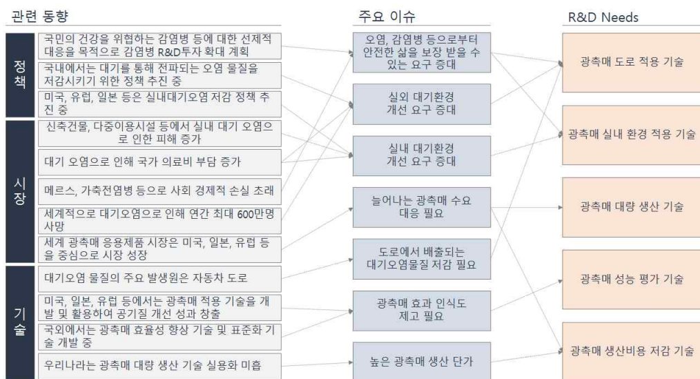
그림 146. Issue-Tree 분석
