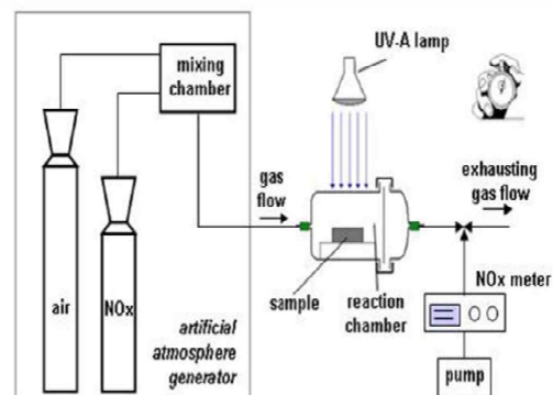
그림 73. CEN/TC386/WG2 시험방법
