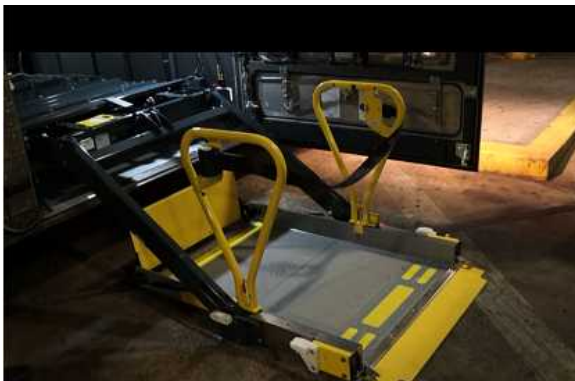
<승강장치 지면위치 하강>
