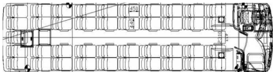
<그림 26> 자일대우 FX120 좌석배치 (42인승)
