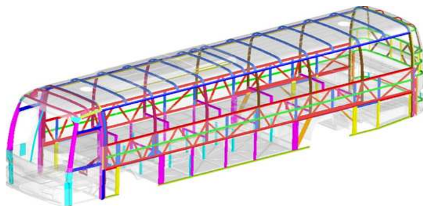
<그림 21> 기아 뉴그랜버드 차체 프레임 구조
