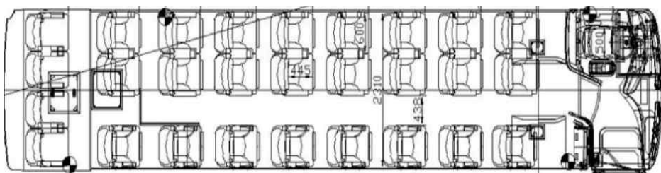
<그림 25> 자일대우 FX120 좌석배치 (29인승)
