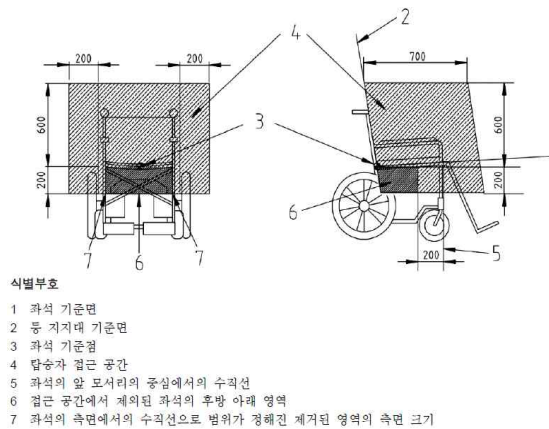
<그림 29> 탑승자 접근 공간
