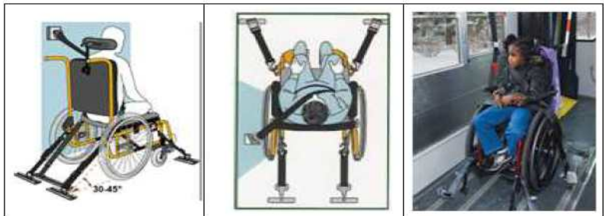
<그림 59> 휠체어 고정장치 기준 관련 자료
