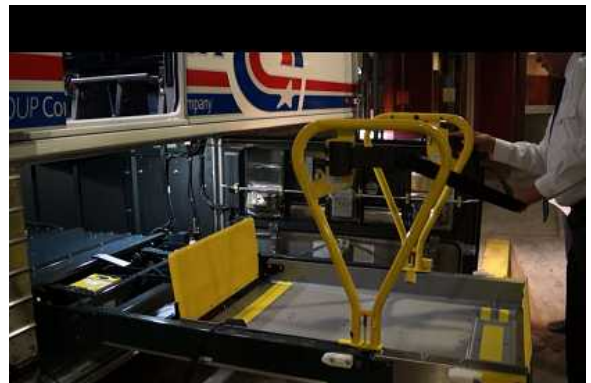
<휠체어 승강장치 돌출>
