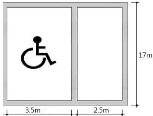
<그림 117> 휠체어 승강장치 사용 필요공간 (교통약자 지역 간 이동실태 연구, 2014)
