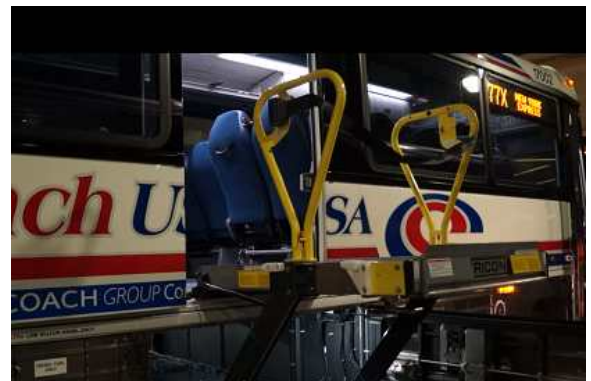
<승강장치 차실위치 상승>
