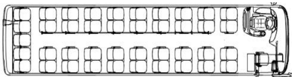
<그림 20> 현대 유니버스 좌석배치 (43인승)
