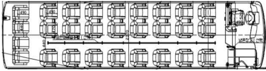
<그림 22> 기아 뉴그랜버드 좌석배치(29인승)
