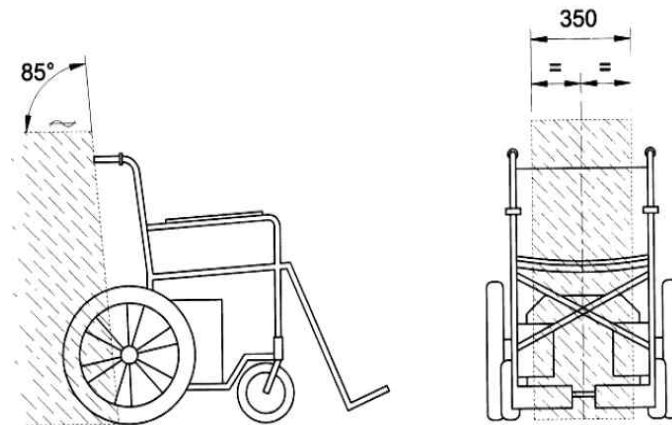
<그림 31> 보호자 이동을 위한 공간
