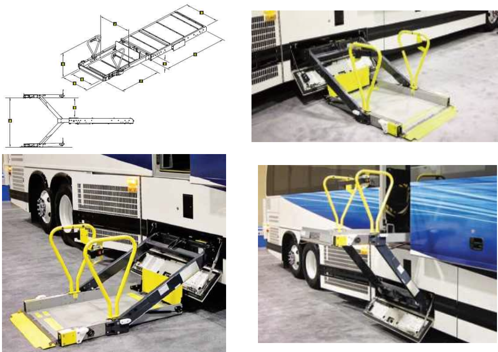
<그림 38> 라이콘사의 매립형 접이식 휠체어 승강장치
