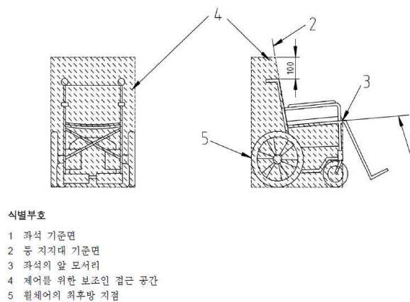
<그림 30> 제어를 위한 보조인 접근 공간
