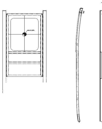
<그림 43> 문틀 설계 및 제작
