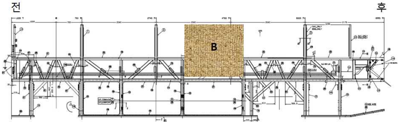
<그림 40> 승강구 개조 위치 선정
