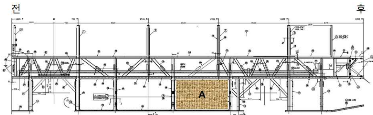
<그림 39> 휠체어 승강장치와 차체구조를 고려한 모듈화 기술
