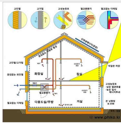
그림 1 Passive House 개요
