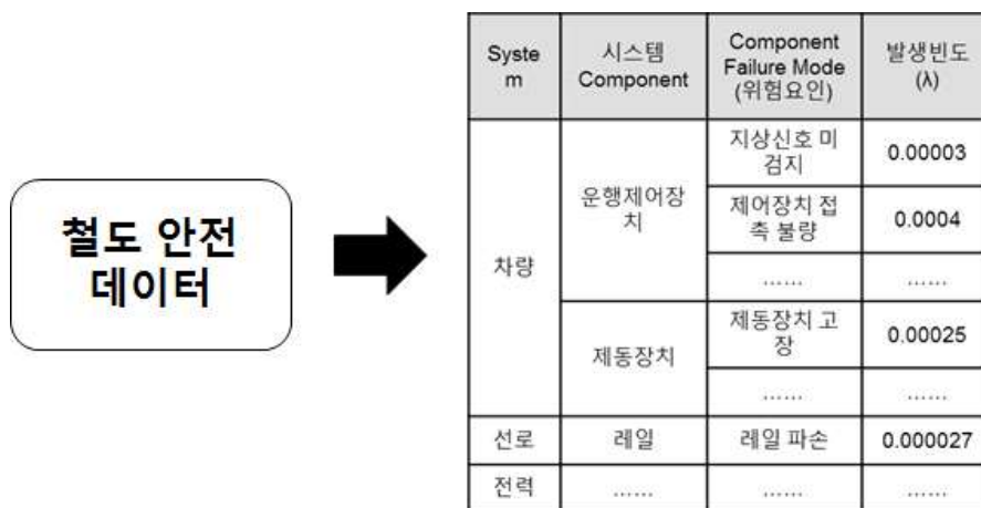
그림 92. 위험요인의 발생빈도 산출 예시
