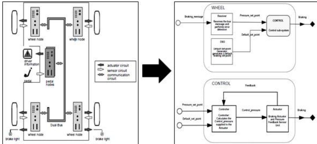
그림 82. 시스템 파악 예시, Hierarchical Modeling of braking wire system (Papadopoulos, 2000)
