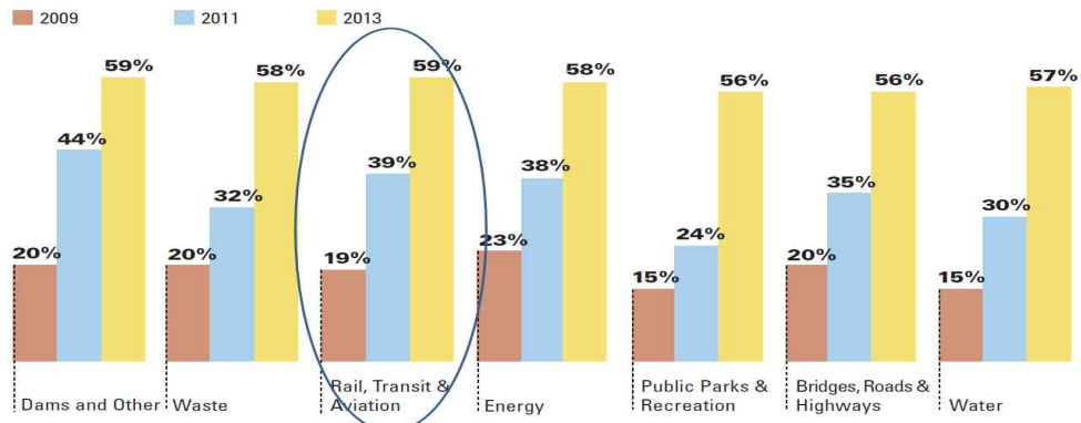
그림 78 미국 토목인프라분야에서의 BIM 적용, McGraw-Hill Construction, 2012
