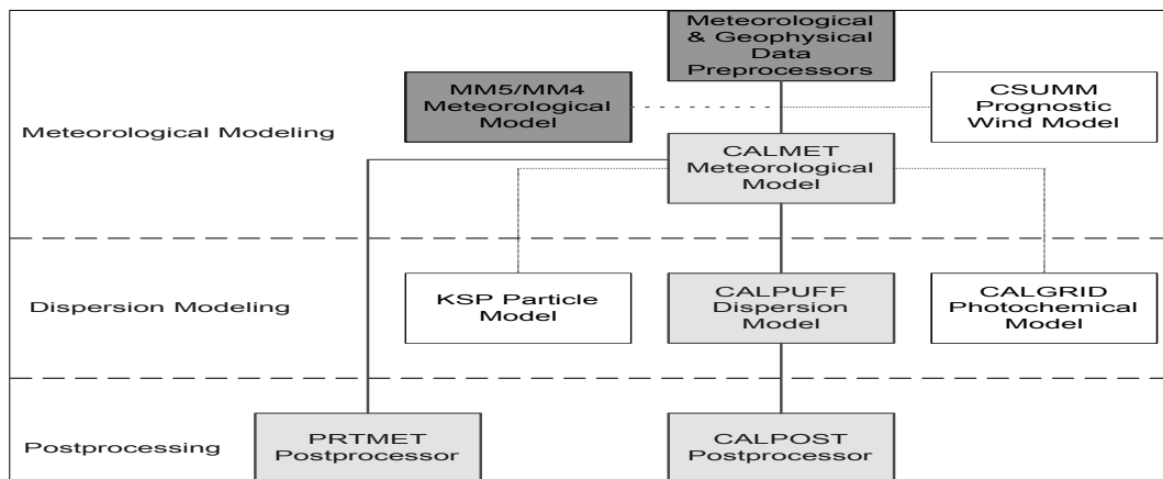
<그림 5-21> CALPUFF 모델링 시스템
