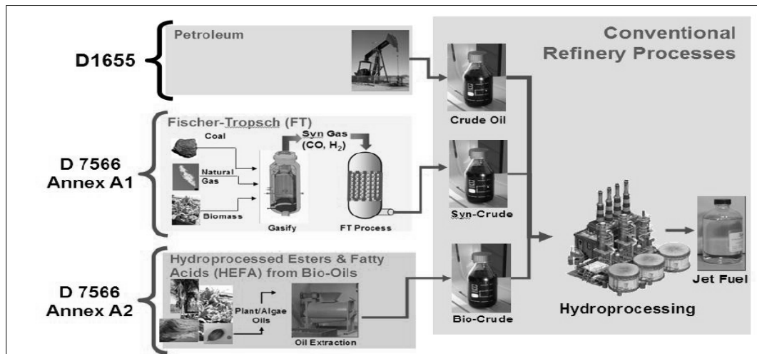
<그림 2-16> F-T 기술 및 HERA 기술 pathway
