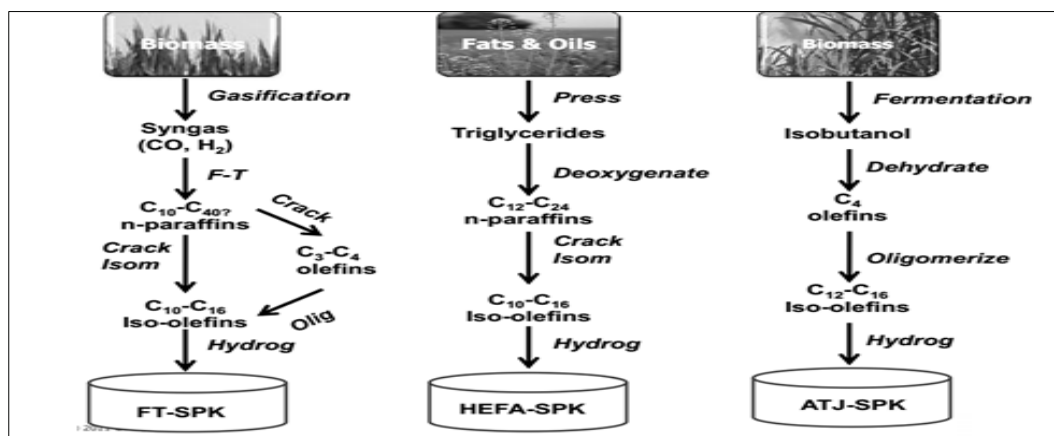
<그림 2-12> 항공용 바이오연료 세부 기술
