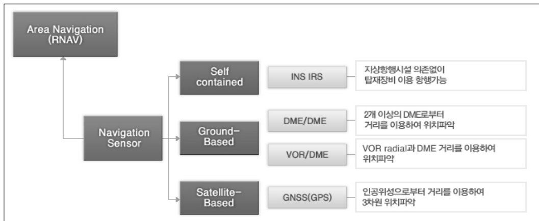
<그림 1-4> RNAV 성능을 제공하는 항행시스템
