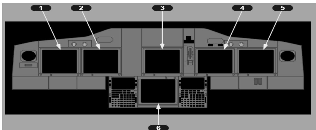
<그림 4-14> B737용 조종석 PFD/ND 디스플레이 예상 배치도
