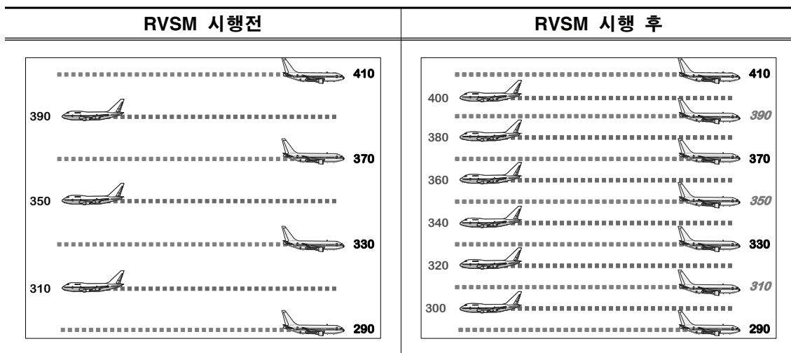
<표 1-1> RVSM 개념도
