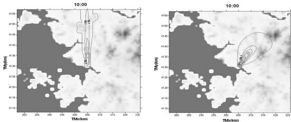
<그림 5-22> 점오염원에 대한 ISCST3와 CALPUFF 모델 결과
