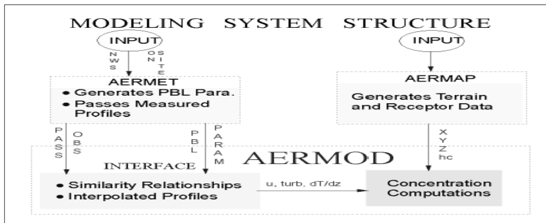
<그림 5-20> AERMOD 구성도
