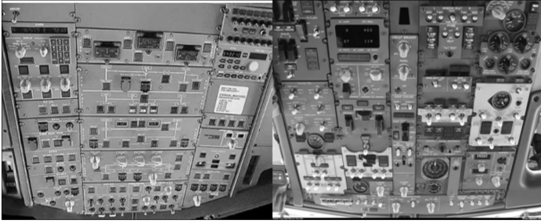
<그림 4-12> 오버헤드 패널 사진(좌: A320, 우: B737)
