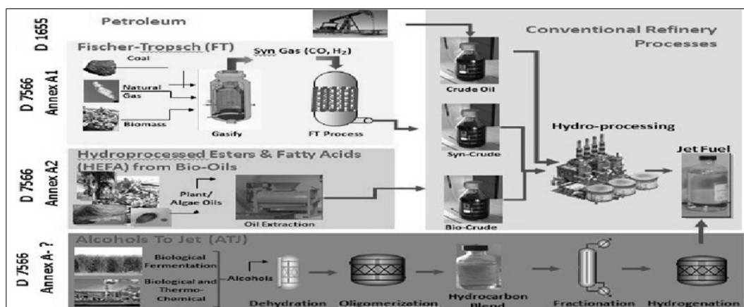
<그림 2-13> 항공용 바이오연료 생산 공정
