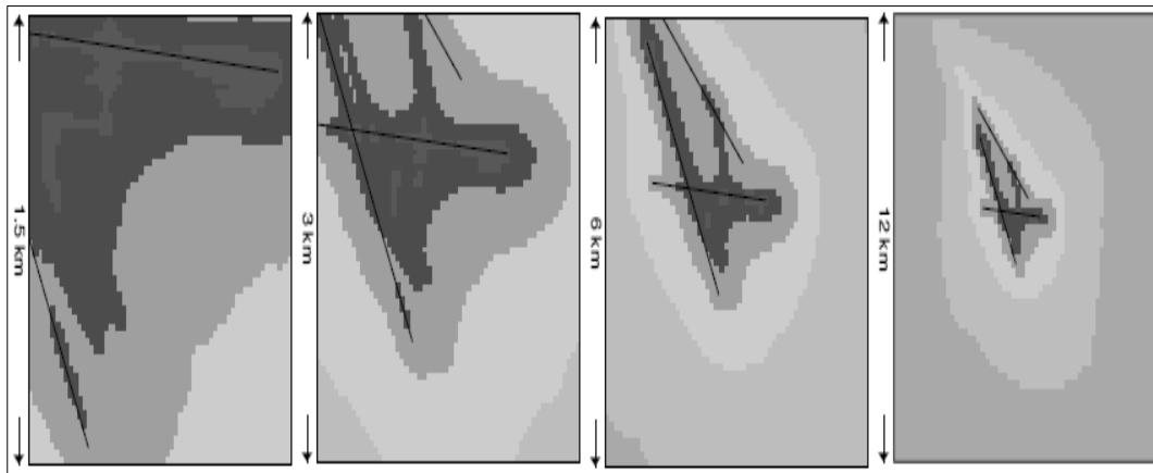
<그림 5-31> LASPORT 적용 NOx 농도 시각화
