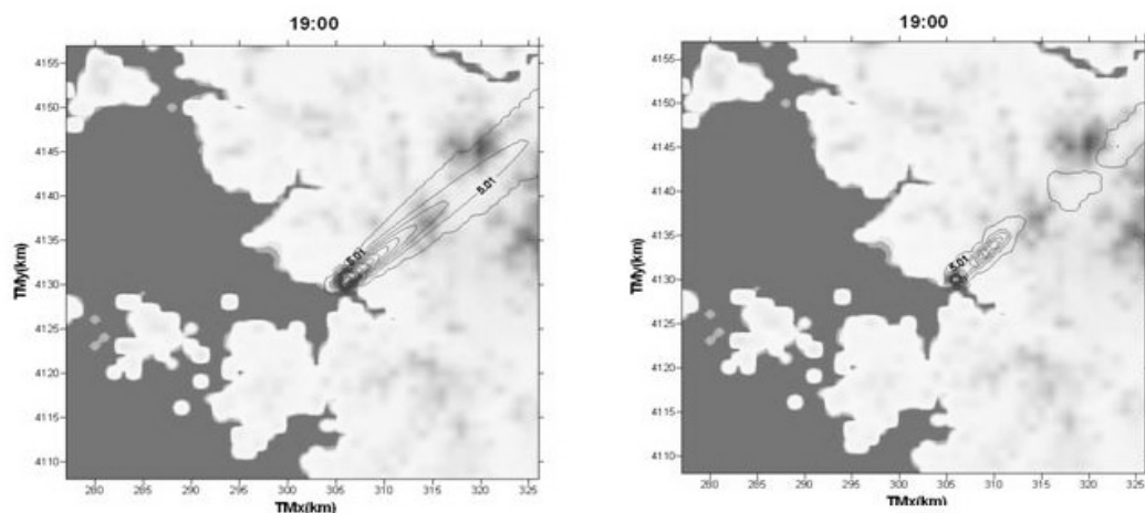
<그림 5-19> AERMOD 대기확산 모의 결과(지형 고려)
