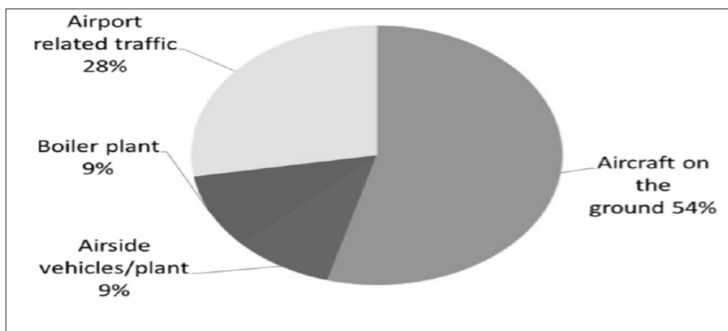
<그림 5-3> 히드로 공항 배출원별 NO 2 배출비중
