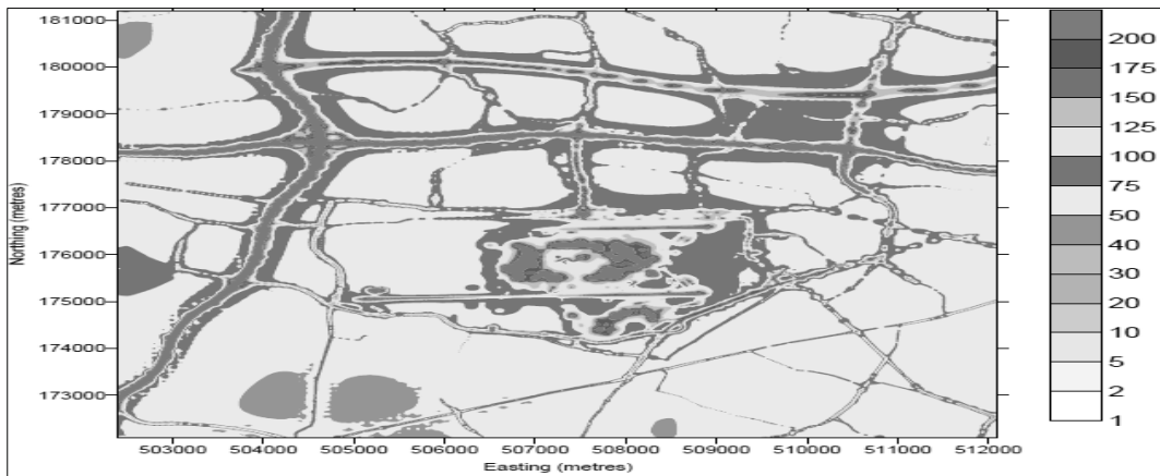
<그림 5-29> ADMS-Airport 히드로 공항 주변 NOx 배출농도
