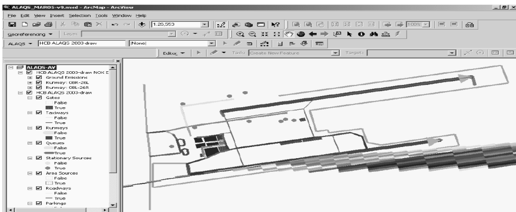
<그림 5-28> ALAQ5-AV NOx 배출농도 결과
