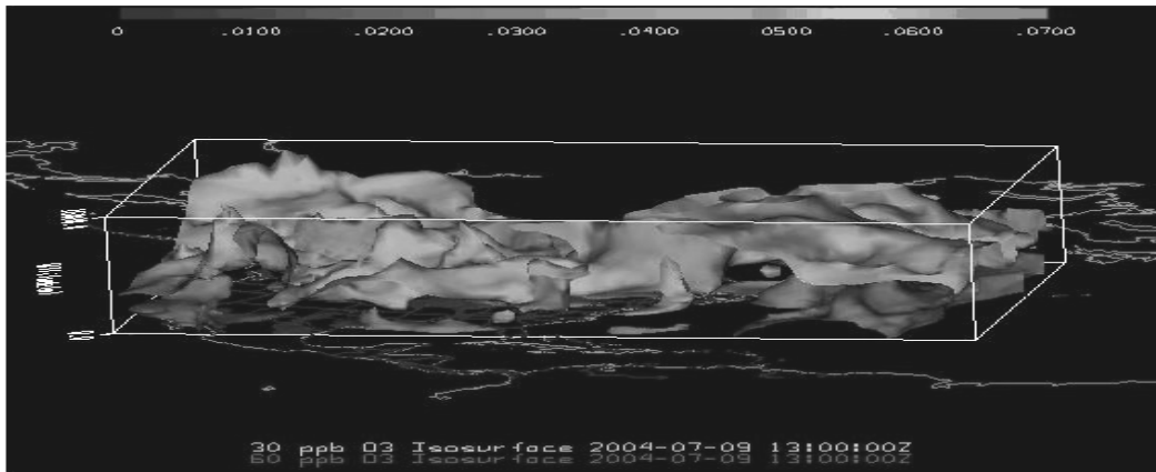
<그림 5-17> CMAQ ver 5.0.1을 통한 오존확산 정도
