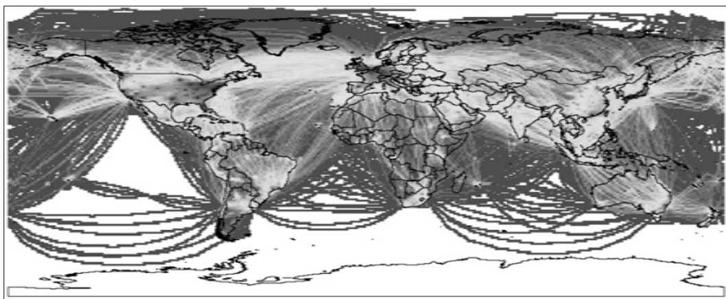
<그림 3-6> AEDT의 출력 결과물: 글로벌 온실가스 배출량 합계
