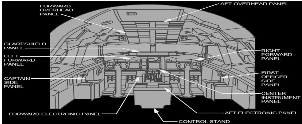
<그림 4-13> 예코플라이트 시뮬레이터 내부 전체예상 배치도
