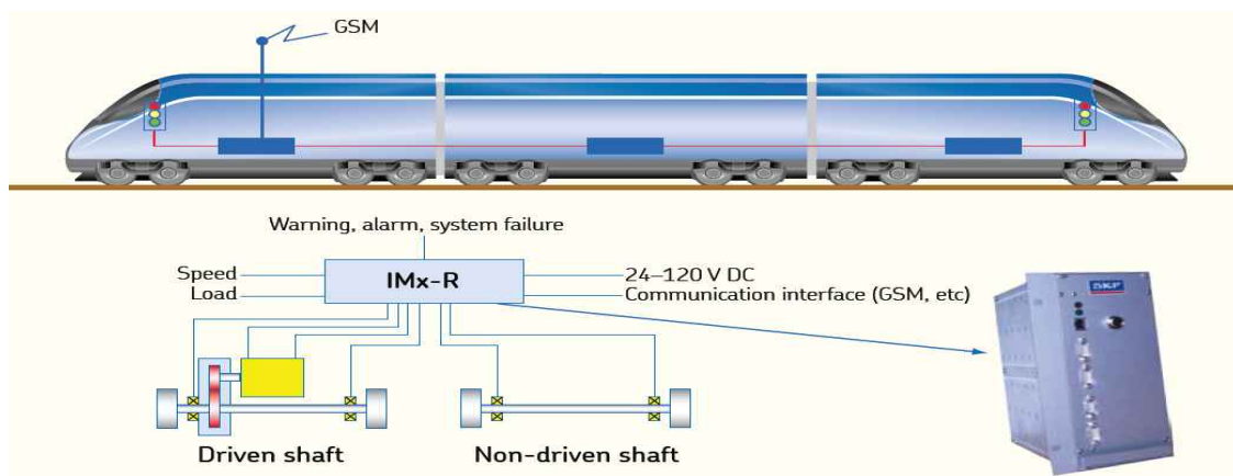
그림 62. Railway bogie condition monitoring 시스템 (SKF)
