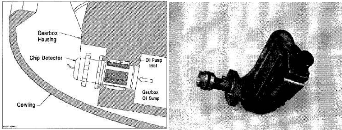
그림 66. 기존 chip detector 방식(좌)과 AH-64 ODM 센서
