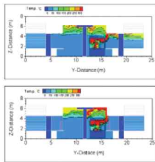
PSD 설치시 상단 내화재 검토 (설치전(상)/후(하)의 유동패턴 변화)
