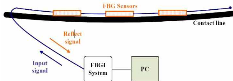
그림 52. FBG 센서를 활용한 전차선 모니터링 시스템 구성
