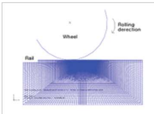
〈WEL 두께변화에 따른 접촉피로 수명평가〉
