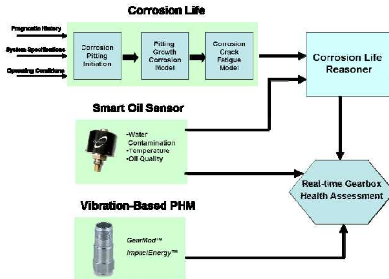
그림 65. 통합형 기어박스 모니터링 시스템
