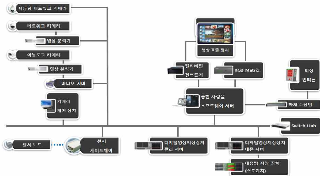
그림 77. 지능형 종합감시시스템 표준 구성도
