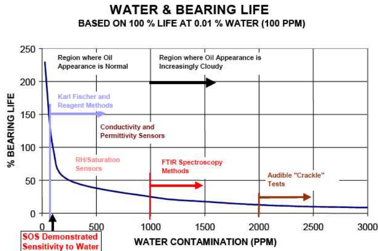
그림 64. 베어링 수명에 미치는 수분함유량의 영향
