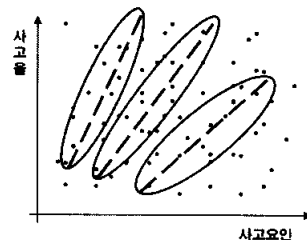
(CART분석모형의 장점)
