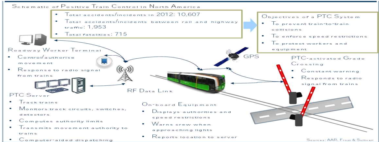
그림 13. Schematic of Positive Train Control(PTC) System (North America)
