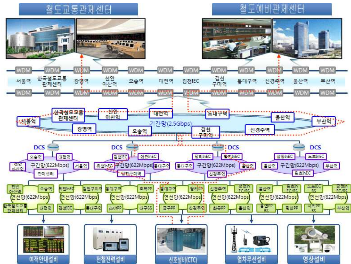
그림 24. 철도 전송망 구성도
