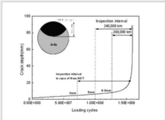
〈균열깊이에 따른 유지보수 주기 설정〉
