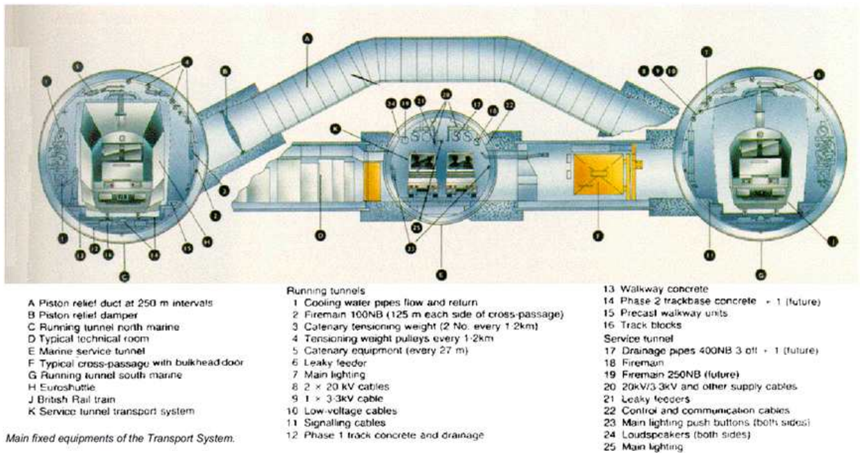
그림 74. 영불유로터널 방재시스템 및 통합 관제실 설치 사례
