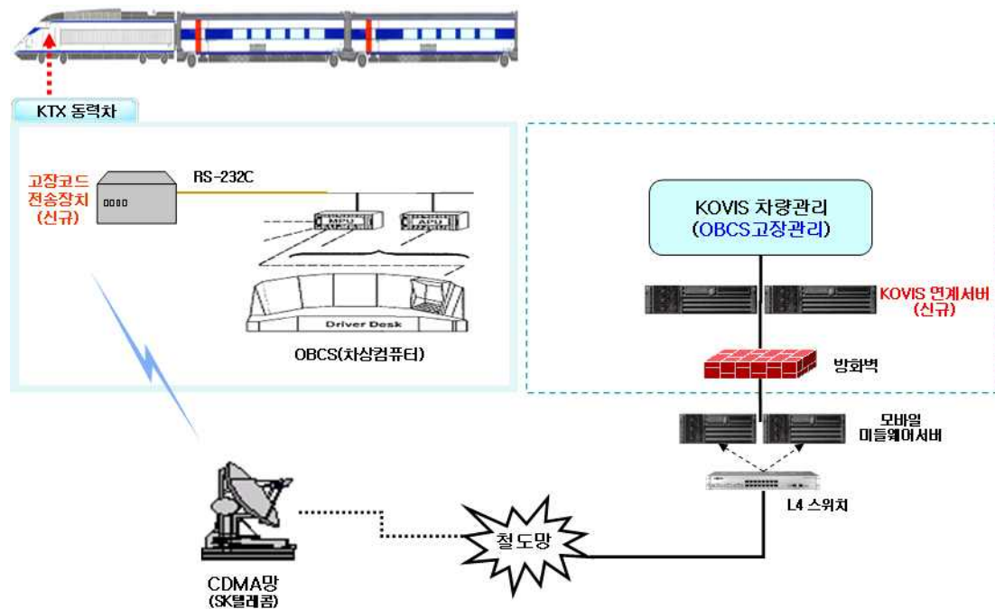
그림 49. 고장코드 무선전송 시스템 구성도
