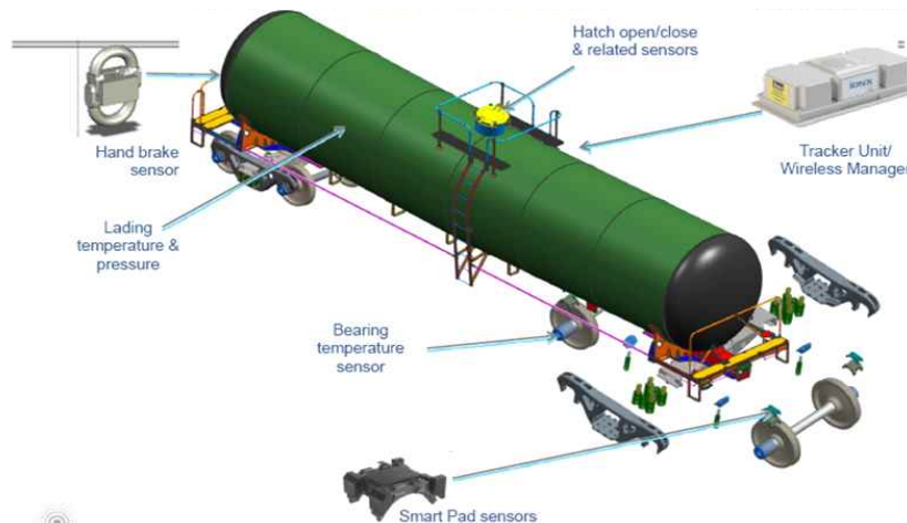
그림 59. INOX Product Placement (Amsted 社)
