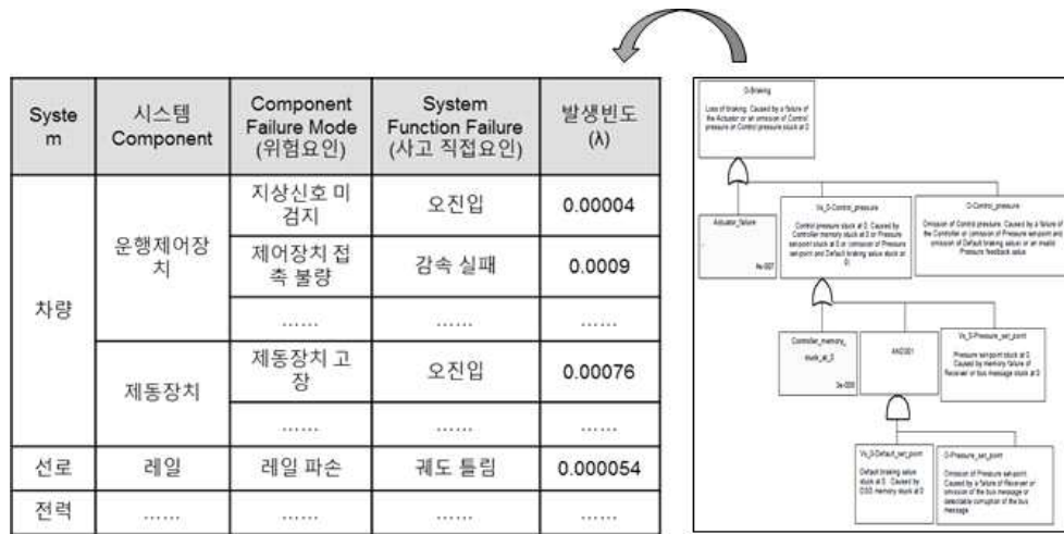
그림 93 직접요인의 발생빈도 산출 예 및 FTA 예시
