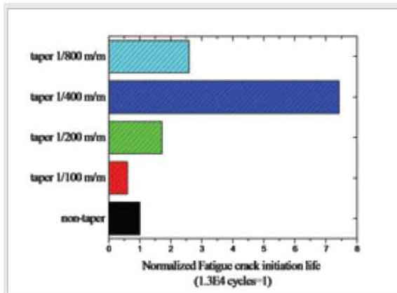
〈테이퍼에 따른 피로균열 발생수명의 변화〉
