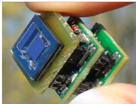
그림 60. 완전 자가발전 무선 온도센서
