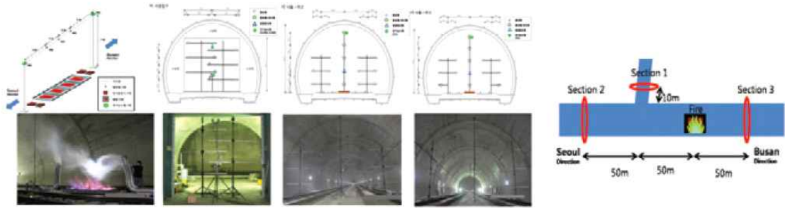
터널 현장화재시험 시스템 개발 내용 및 적용사진 (좌로부터, 화원, 단면1, 단면2, 단면3, 측정시스템)
