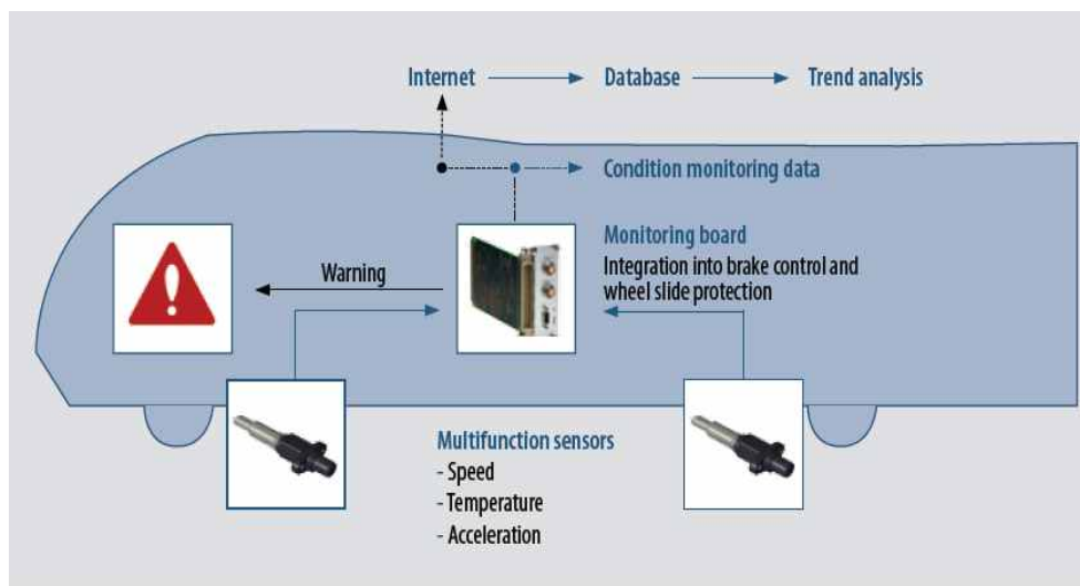
그림 61. 철도차량 대차 모니터링 진단시스템
