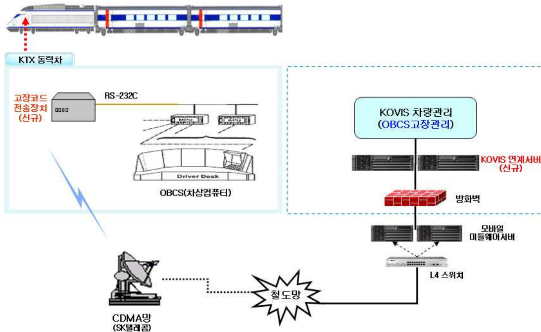
그림 23. KTX 고장코드 무선전송 시스템 구성도
