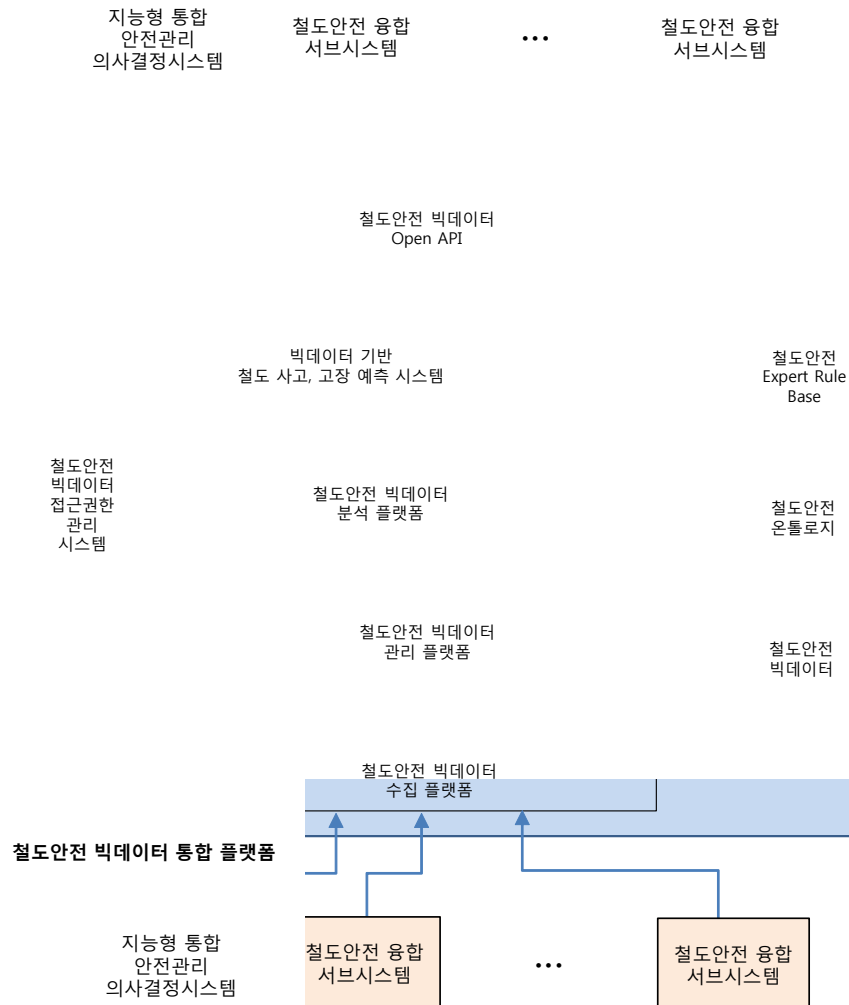
그림 119. 철도안전 빅데이터 통합 플랫폼 구조도
