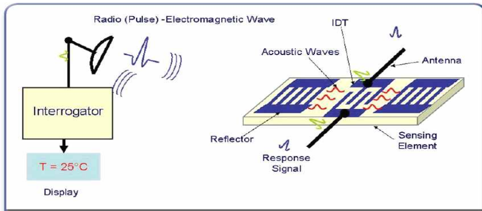
그림 63. SAW 센서를 이용한 무선 온도 계측 시스템
