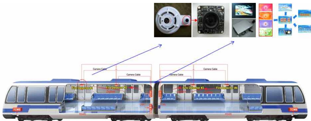
그림 71. 철도차량용 지능형 화재감지시스템 [(주)이플러티, 2010]
