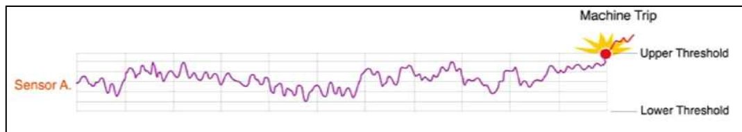
그림 35. 이상징후 판단(예)
