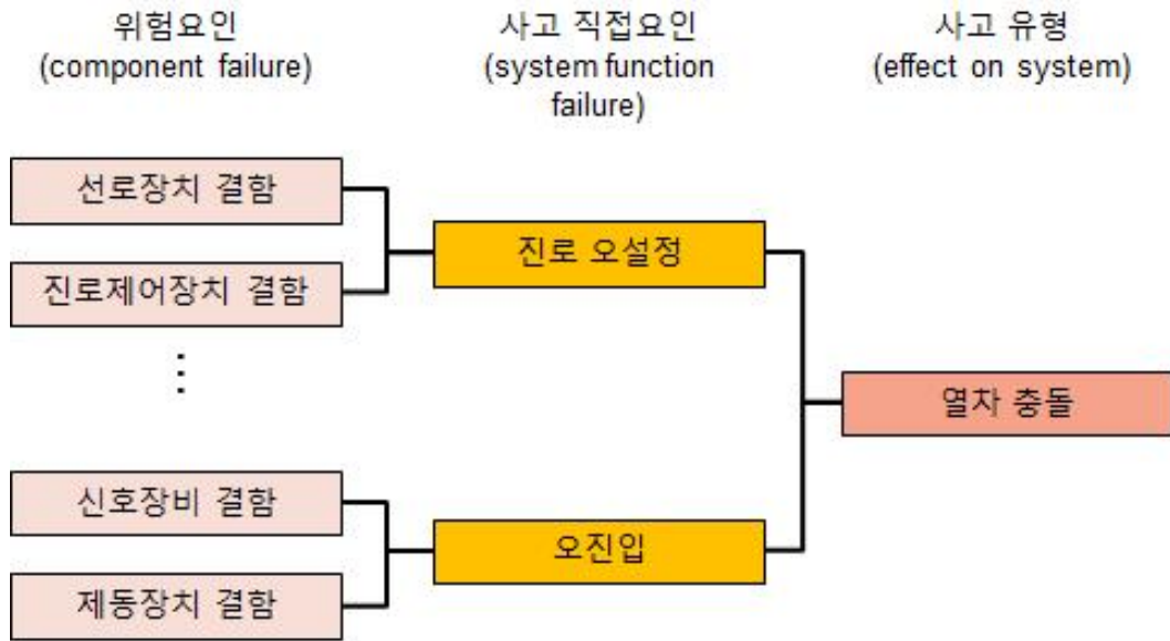
그림 86 사고 유형별 사고 시나리오 도출 예시
