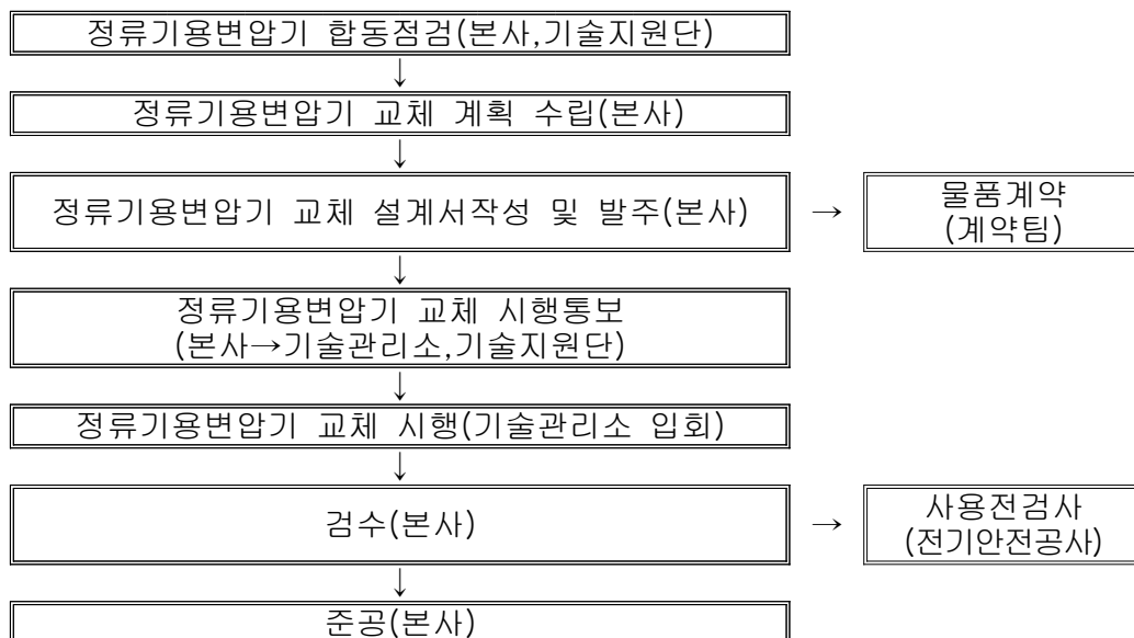
<그림2-21> 서울도시철도공사 정류기용 변압기 교체업무 프로세스
