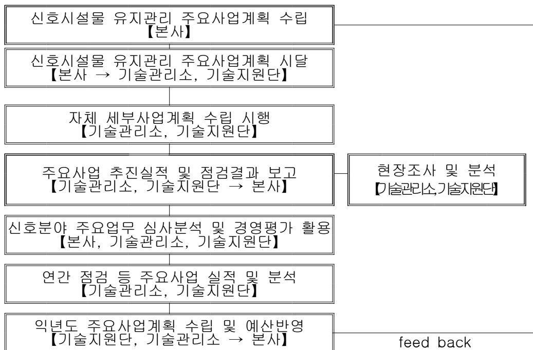
<그림2-23> 서울도시철도공사 신호분야 유지관리 프로세스
