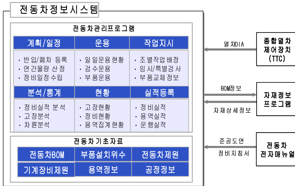
<그림2-39> 광주도시철도공사 전동차 유지보수 프로세스
