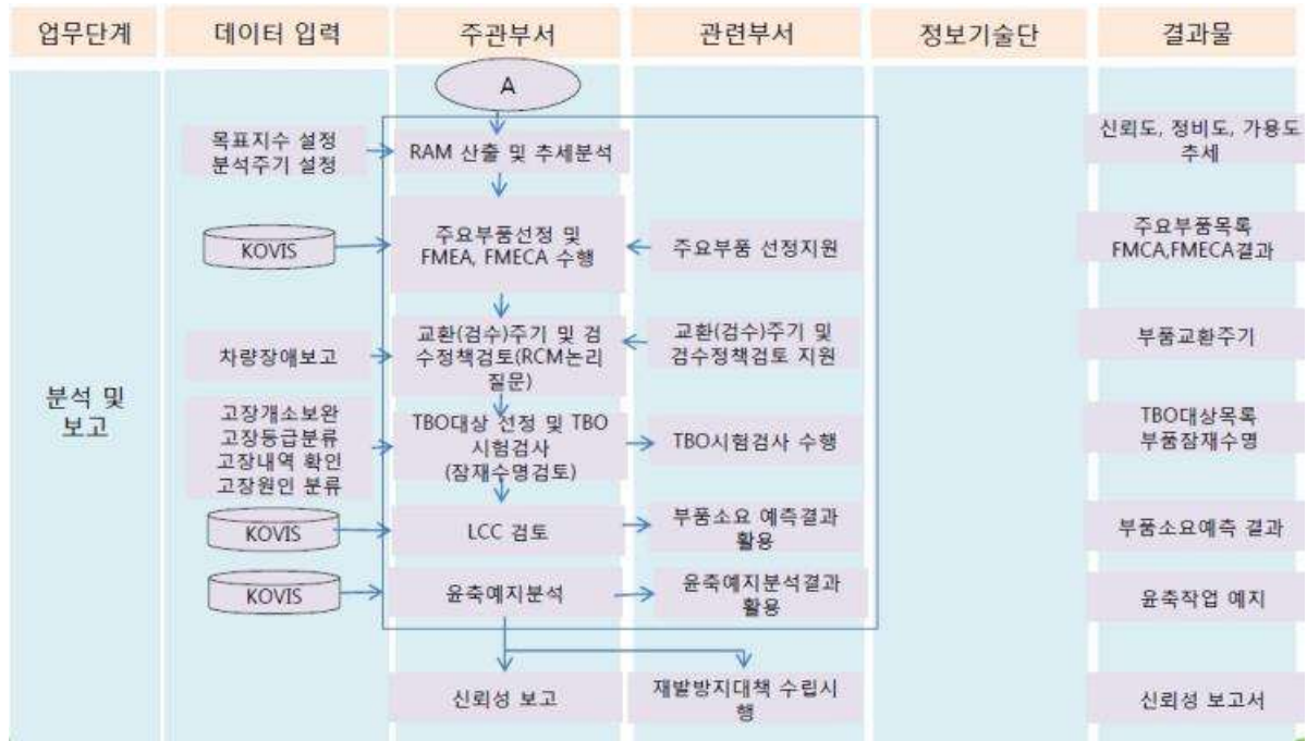
<그림6-4> 분석 및 보고 단계 프로세스
