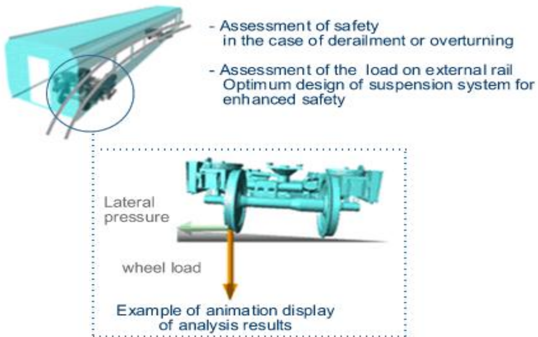
<그림6-11> Hitachi Dynamic Simulator
