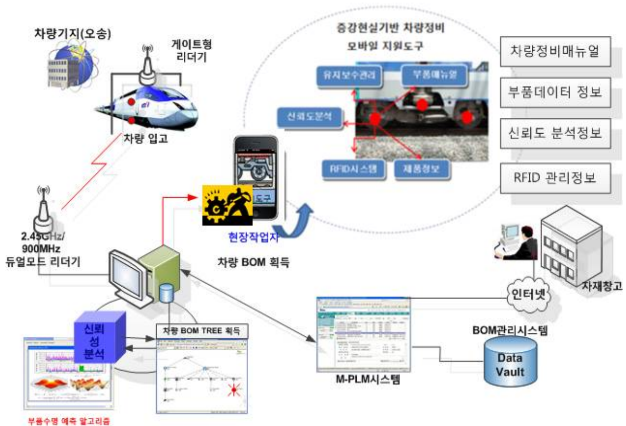
<그림6-18> 유지보수 지원용 모바일 플랫폼
