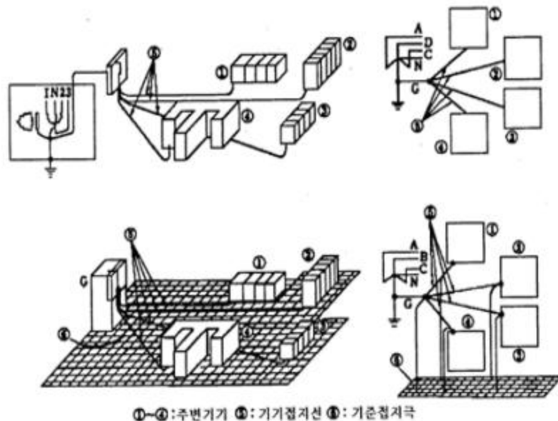
<그림6-23> 다점 접지시스템 구성
