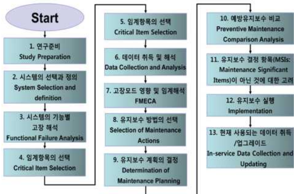
<그림2-65> RCM(신뢰도 중심정비)수행절차
