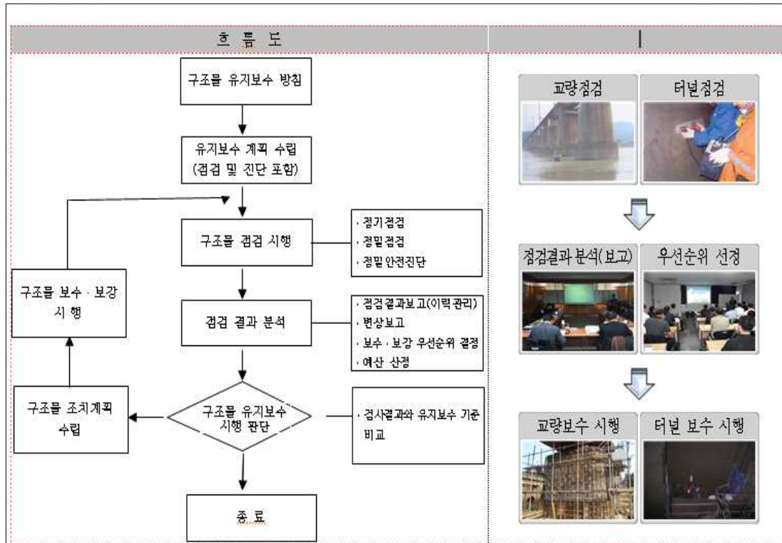
<그림2-5> 철도 구조물 유지보수 업무체계
