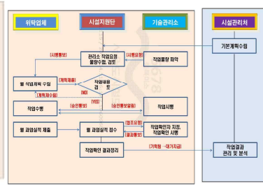
<그림2-26> 서울도시철도공사 궤도분야 유지관리 프로세스
