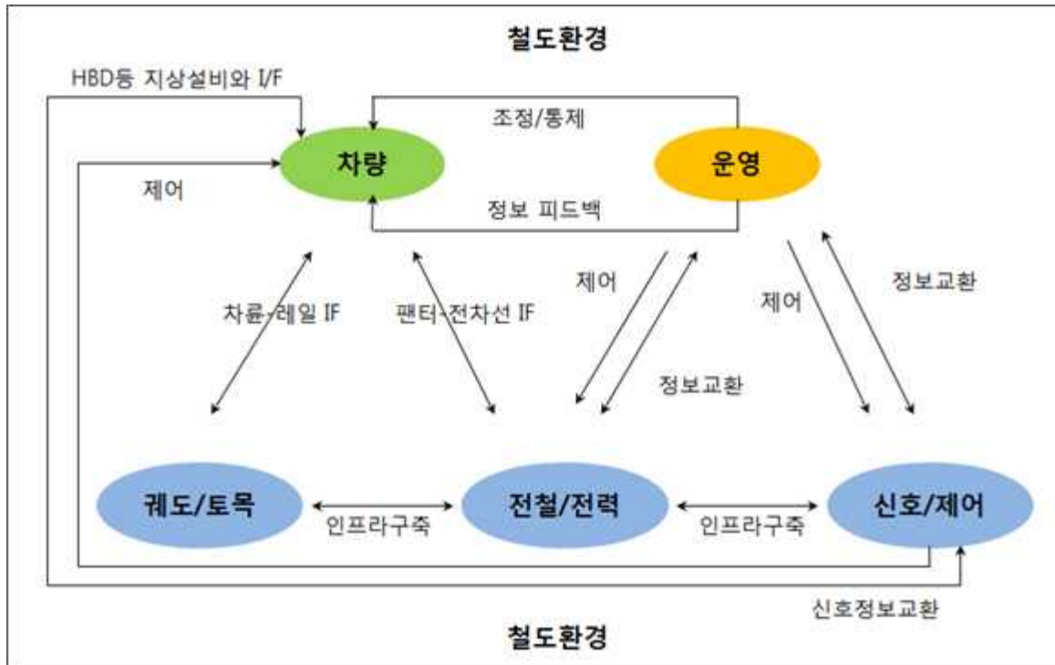
<그림1-1> 철도 운영 및 유지보수 인터페이스
