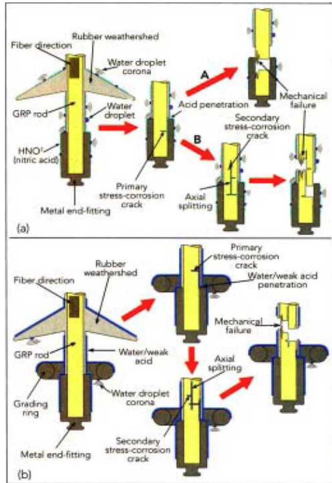
<그림6-22> 폴리머매자 취성파괴 메카니즘
