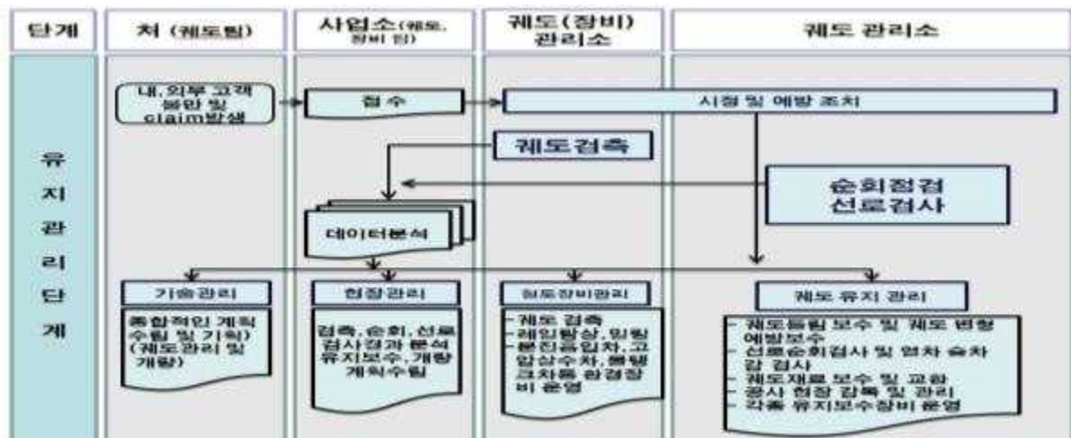
<그림2-15> 서울메트로 궤도 유지보수 업무 체계
