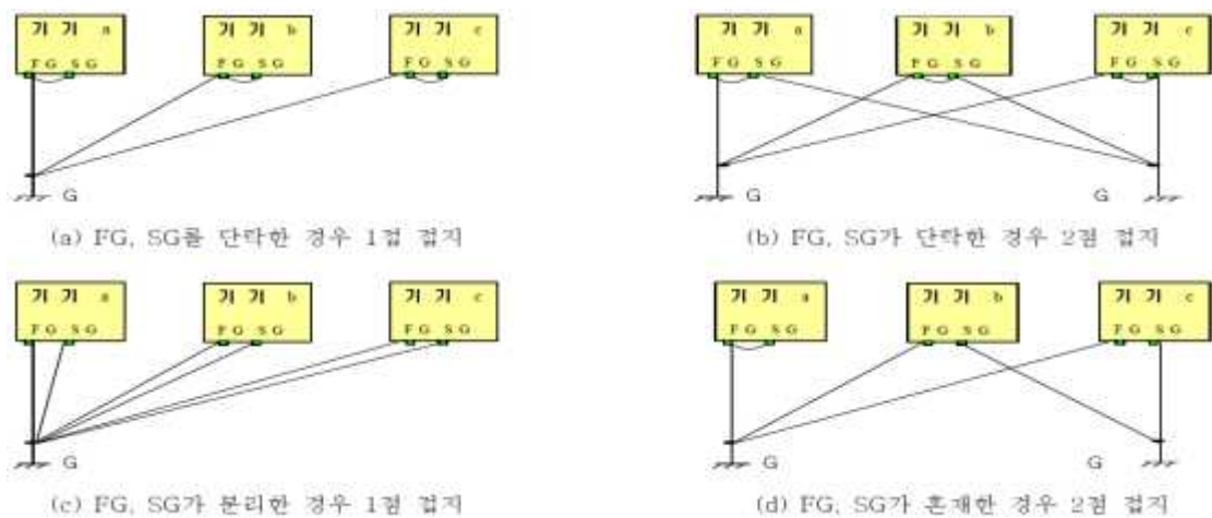
<그림6-25> 접지 공용시 접속상태
