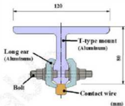
<그림6-27> T-bar 강체 단면
