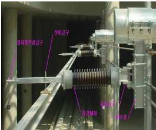
<그림6-28> R-bar 가선방식
