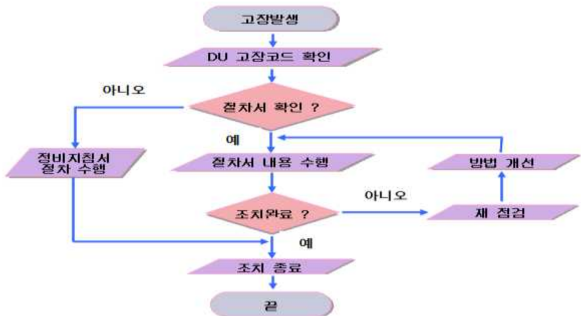
<그림2-40> 광주도시철도공사 전동차 고장조치 프로세스
