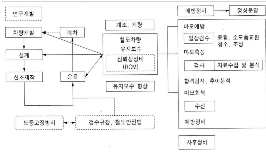
<그림2-3> 철도차량 유지보수 업무체계
