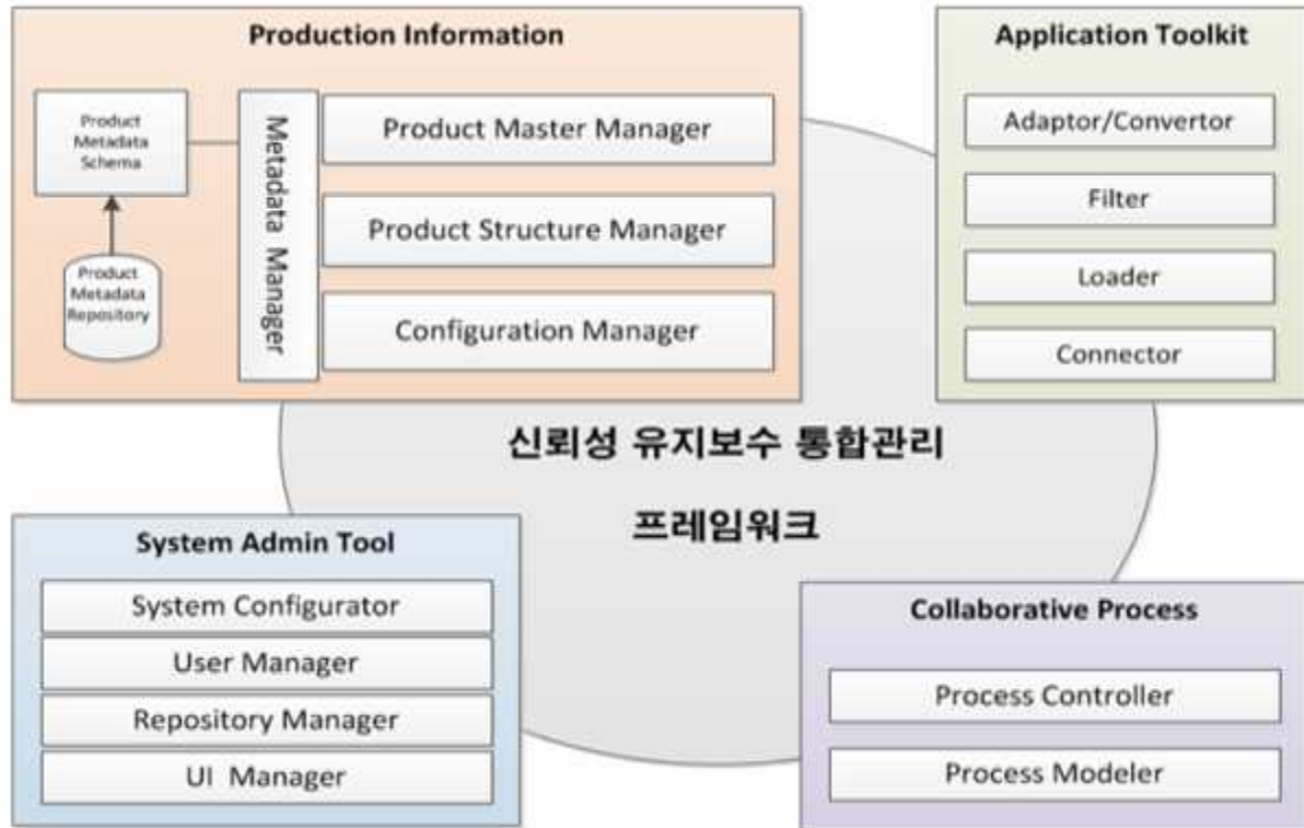
<그림6-15> 신뢰성 기반 유지보수 통합관리 프레임워크
