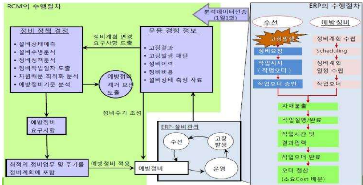
<그림6-2> KTX-RCM 업무 흐름도
