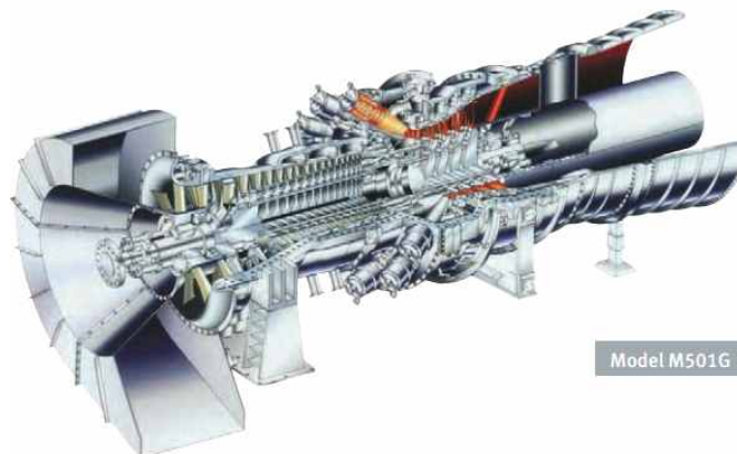
그림 56 두산중공업 가스터빈엔진(M501G)
