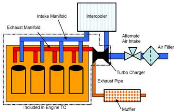
그림 135. Intake system 구성도
