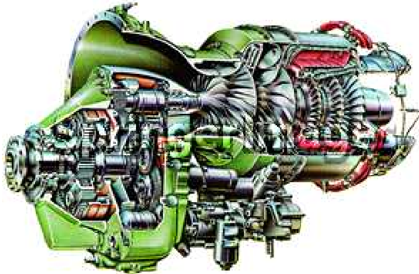
그림 10. Turboprop Engine (Garrett, TPE 331)
