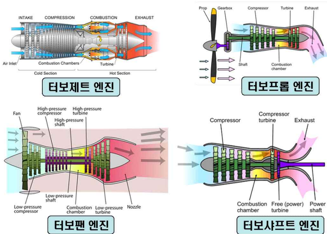
그림 7 가스 터빈 엔진의 종류
