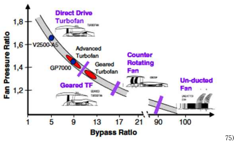
그림 80 항공기 엔진 Bypass Ratio에 대한 Fan Pressure Ratio
