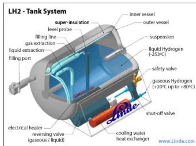
그림 166. Linde사 액체수소 탱크
