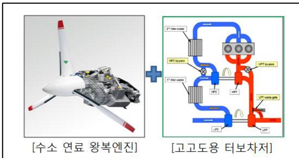
그림 167. 항공기용 수소 왕복엔진 시스템
