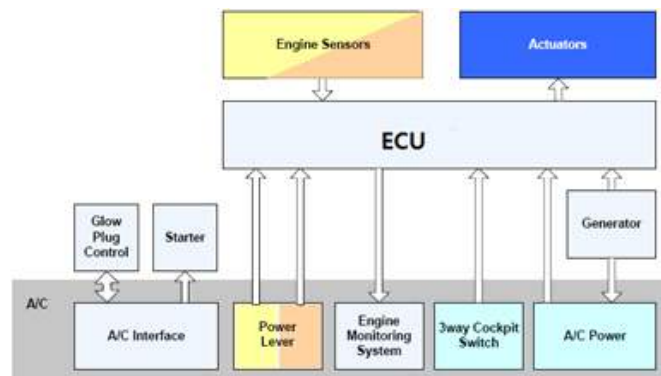
그림 137. ECU 구성도
