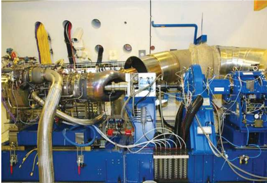
그림 70. KARI 터보 샤프트 엔진 시험 설비
