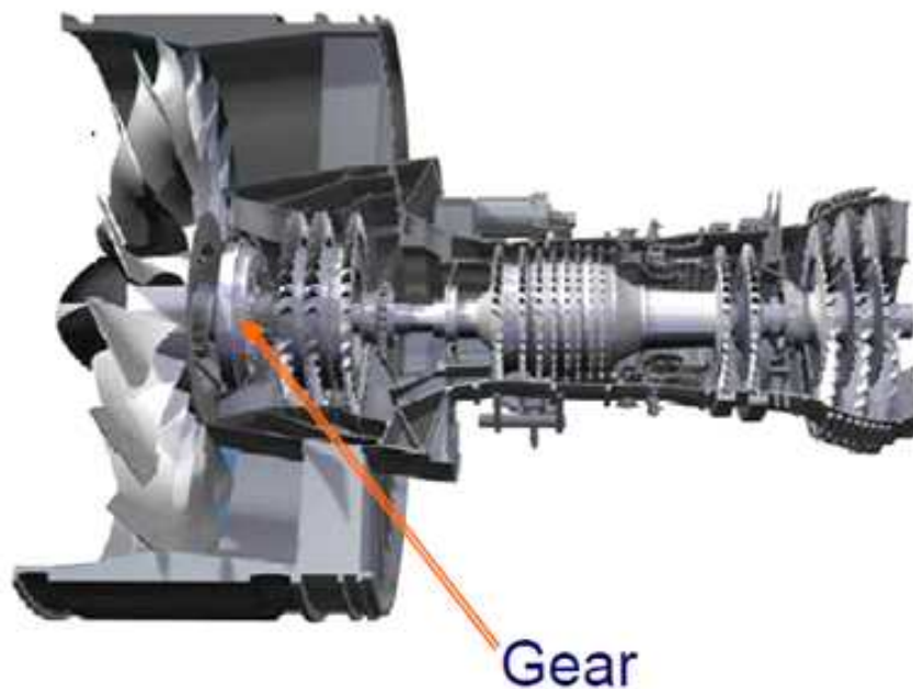
그림 91 PW PurePower Engine
