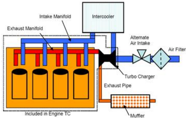
그림 136. Exhaust system 구성도
