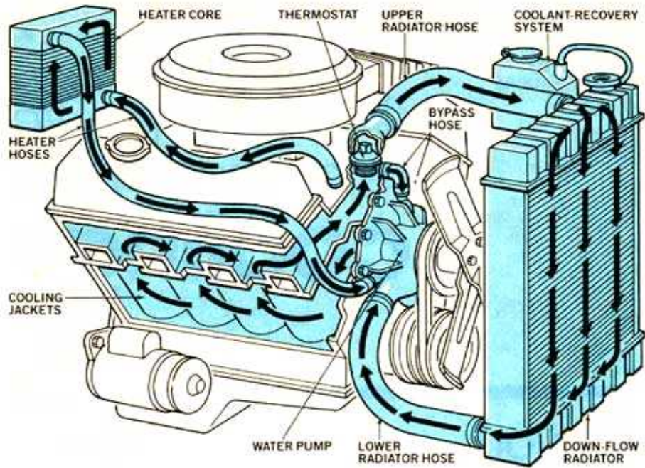
그림 4. 수냉식 엔진
