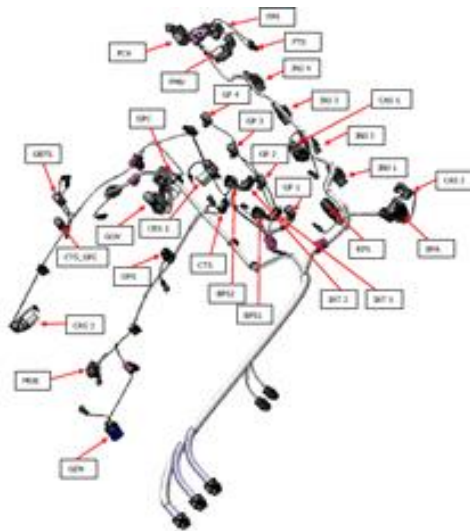
그림 138. Harness 형상
