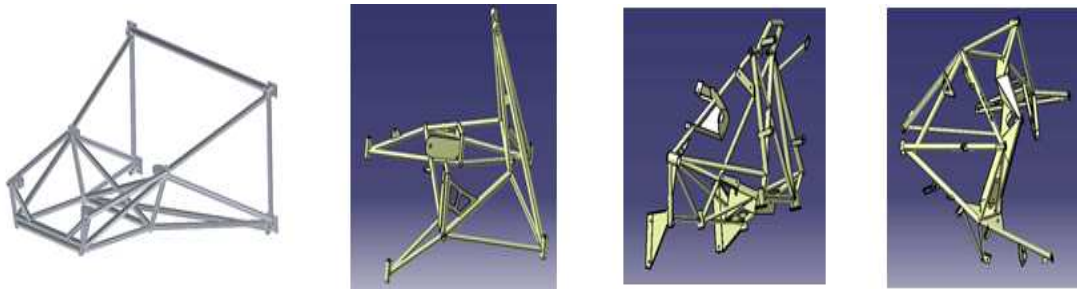
그림 133. 엔진 구조물(예)
