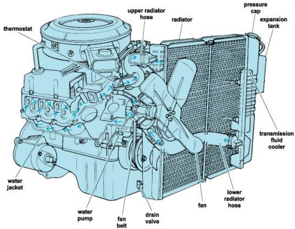
그림 5. 공랭식 엔진
