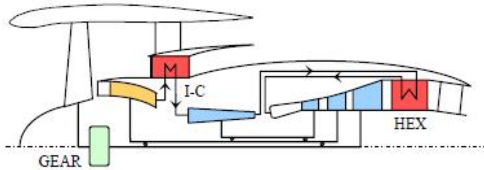
그림 93 Intercooled Recuperative Engine Concept
