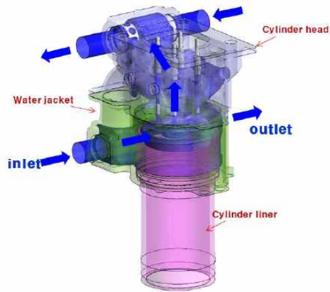
그림 140 열 해석(예)
