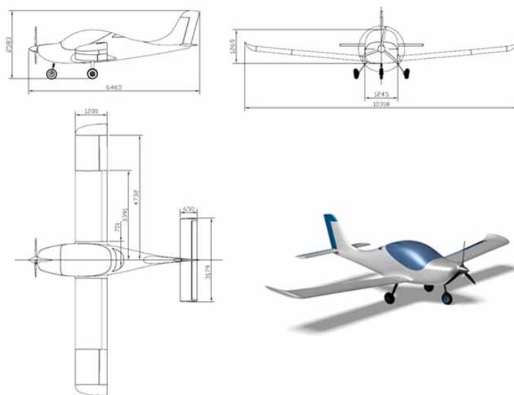
그림 67. KLA-100 삼면도
