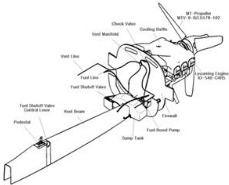
그림 64. 반디호 추진기관 구성도
