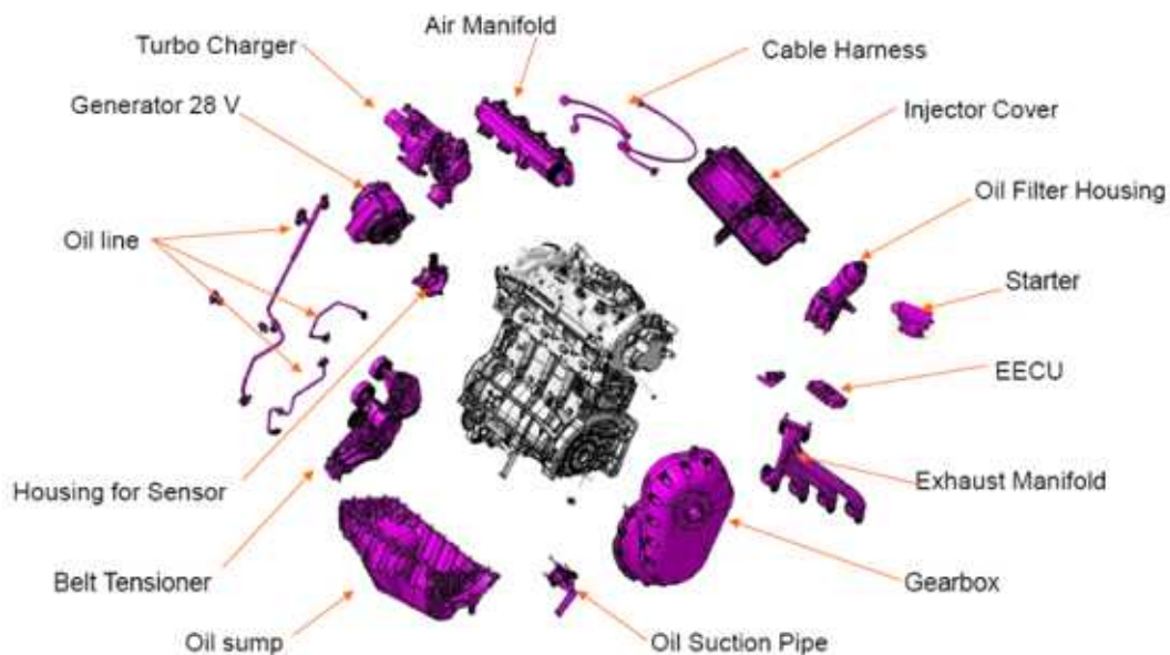
그림 132. 엔진 구성도
