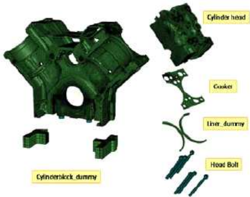
그림 141 구조 해석(예)
