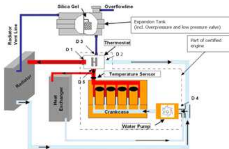
그림 134. Cooling system 구성도
