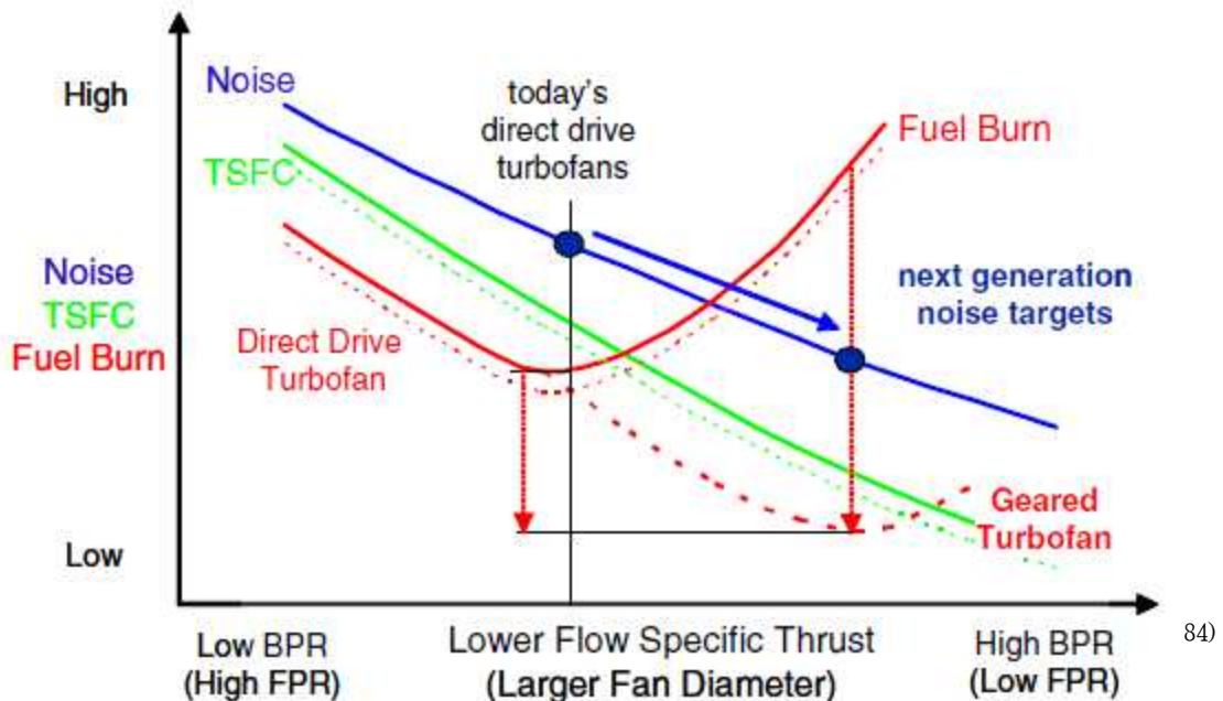
그림 90 Bypass Ratio에 따른 소음, TSFC, 연료연소율 및 소음
