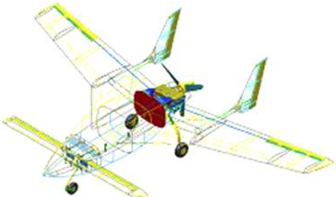
그림 63. 반디호 엔진 장착 개념
