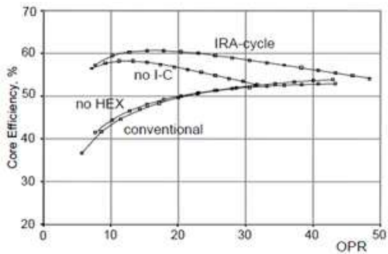
그림 94. I-C, HEX 장착 여부에 따른 효율
