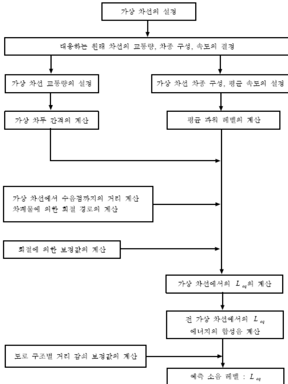
그림 4-38 HW-NOISE 예측 과정
