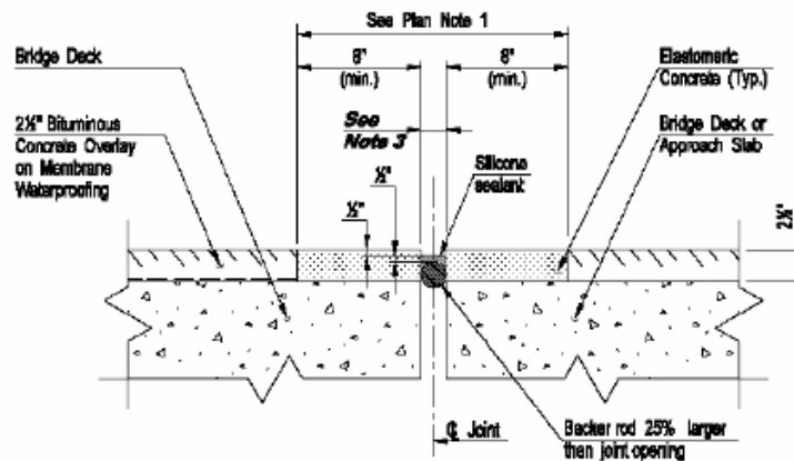
그림 6-9 Elastomeric concrete with silicone sealant
