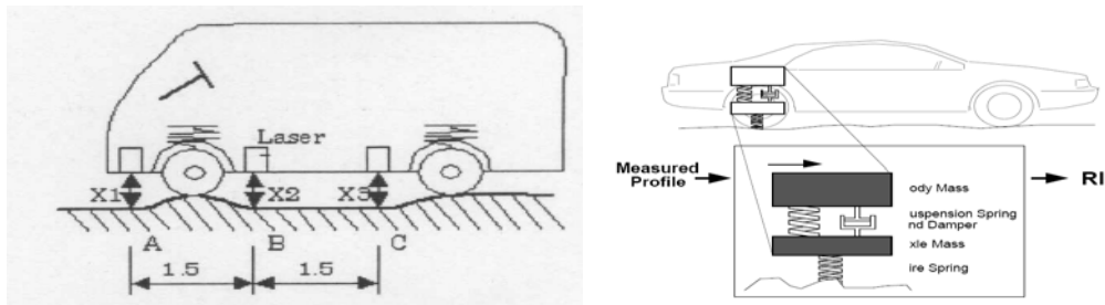
그림 4-46 평탄성 측정 방식(좌: 3점 평탄성 측정방식, 우: Quarter Car Model)
