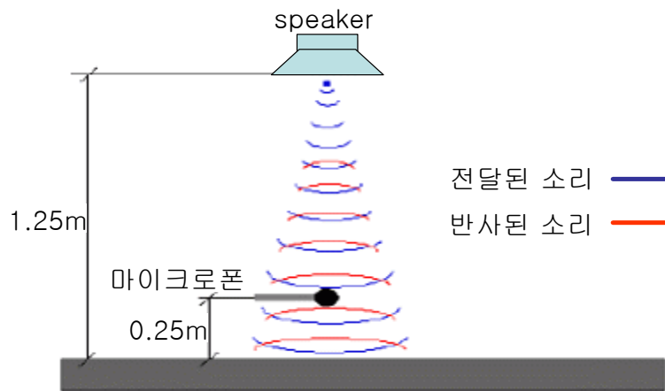
그림 4-35 흡음률 측정 원리(Garai, 1998)
