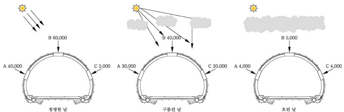
그림 6-40 순응시설내 입사광의 변화
