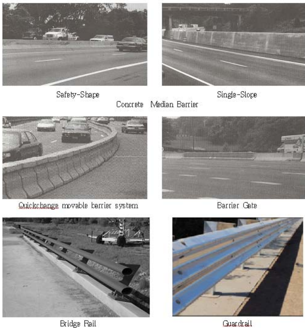
그림 2-7 외국의 종방향 베리어
