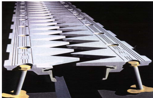
그림 6-12 NEW FINGER JOINT
