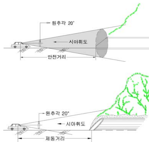
그림 6-34 운전자의 시야휘도 원리
