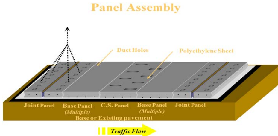
그림 4-6 프리캐스트 슬래브 조립 과정
