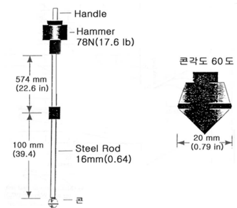
그림 4-13 동적콘관입시험기 개략도
