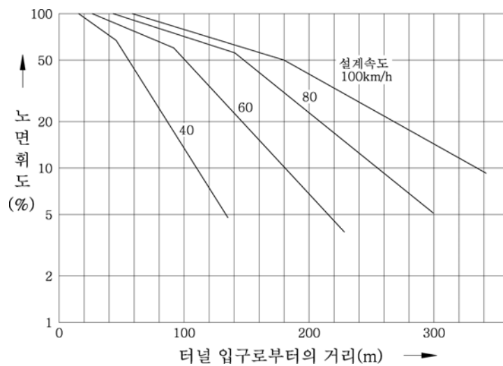
그림 6-43 터널입구부의 노면휘도 (KSA-3703)
