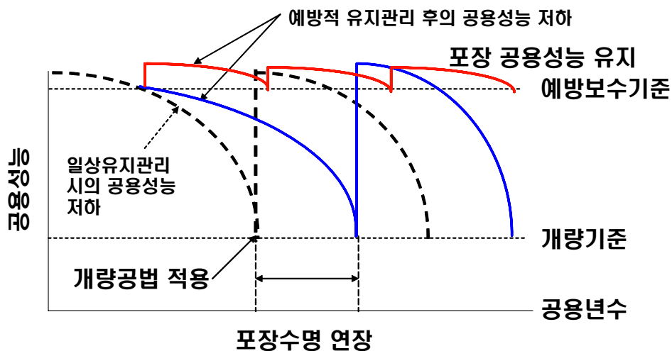
그림 7-6 포장에서의 예방적 유지관리 적용과 포장 성능
