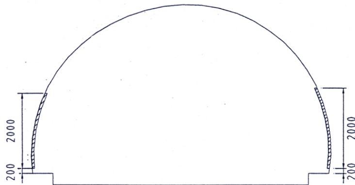
그림 6-32 내장재 세부설치(2m)
