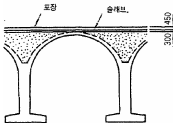
그림 6-20 중복식 아치형 무조인트 방식
