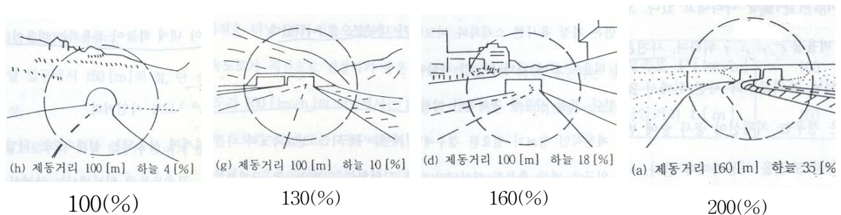
그림 6-35 터널환경에 따른 시야회도의 변화(방위에 따라서도 차이가 있음)
