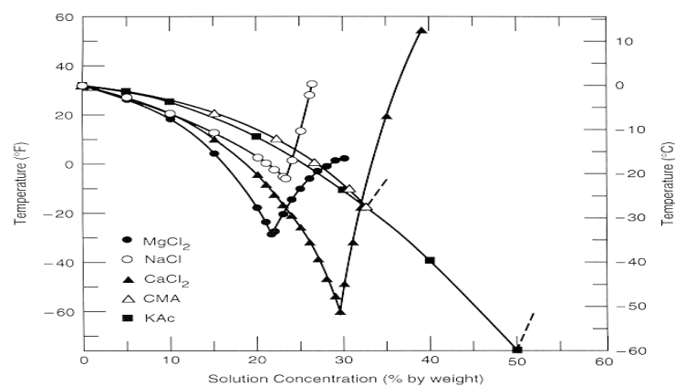
그림 5-22 제설제별 성능 평가
