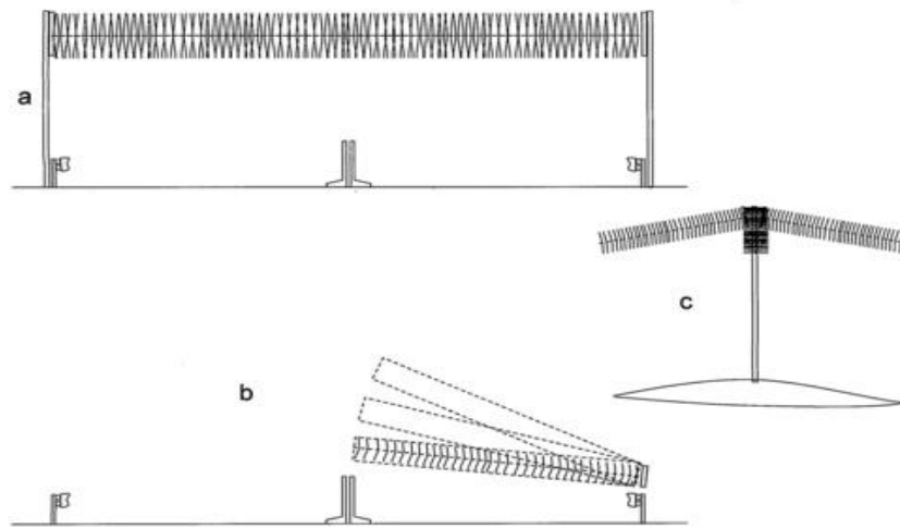
그림 5-6 음파를 이용한 안개제거 장치(Valerio Abete, Italy)
