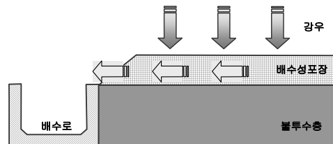
배수로를 통한 배수
