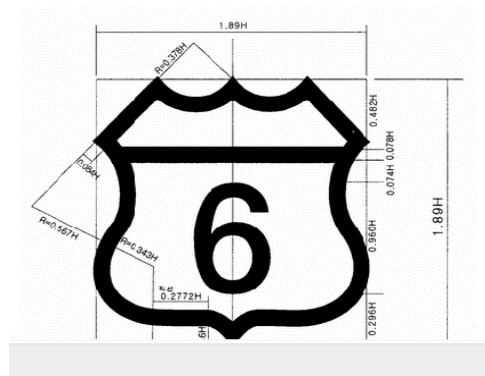
그림 2-16 국내 도로표지판 설계 예
