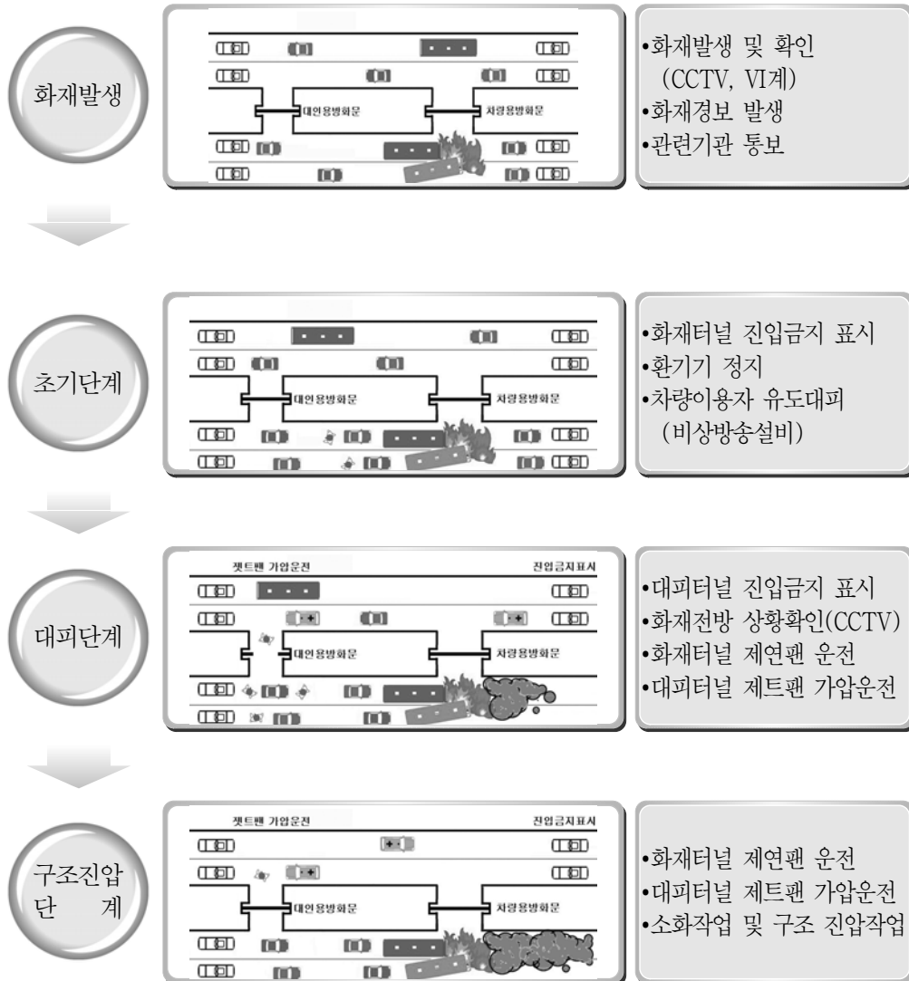
그림 7-14 터널사고 대응 시나리오
