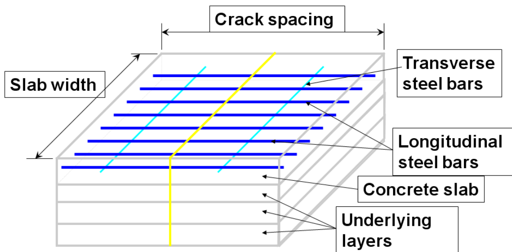
그림 4-5 CRCP 구성도
