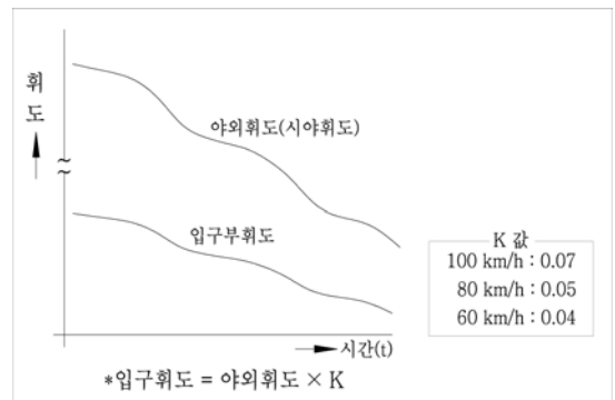
그림 6-38 외부휘도 와 내부휘도 비
