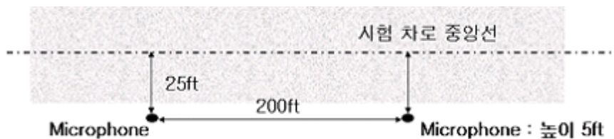
그림 4-24 위스콘신의 단독차량 pass-by method 시험 조건
