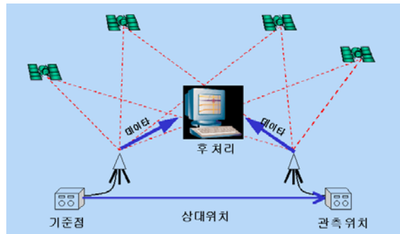
그림 7-8 후처리 상대 측위 기법
