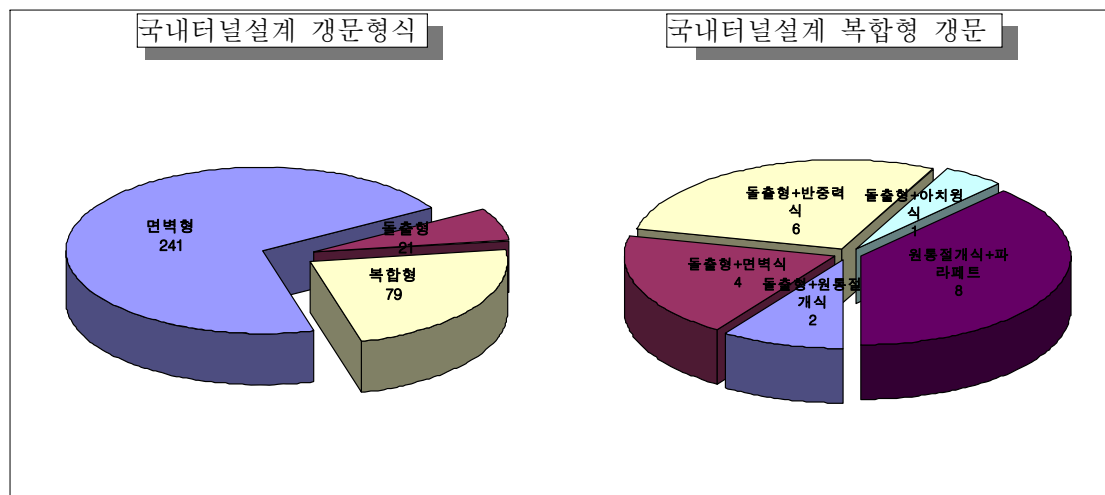
그림 6-24 국내 갭문형식 적용유형
