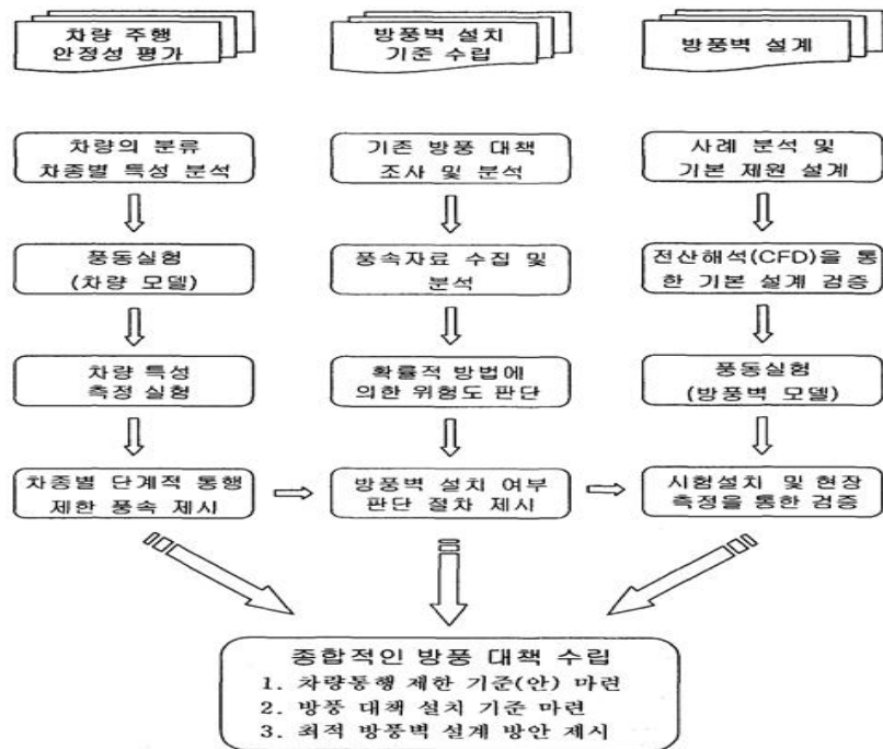
그림 5-5 종합적인 방풍 대책
