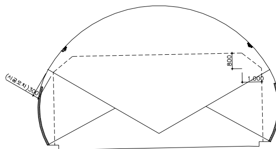
그림 6-27 시공오차 한계
