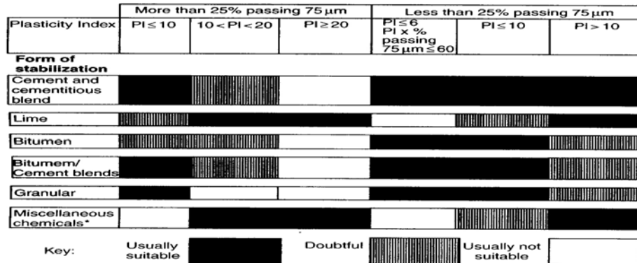
그림 4-17 안정처리 공법의 적용 범위(C.A.O'Flaherty, 2002)
