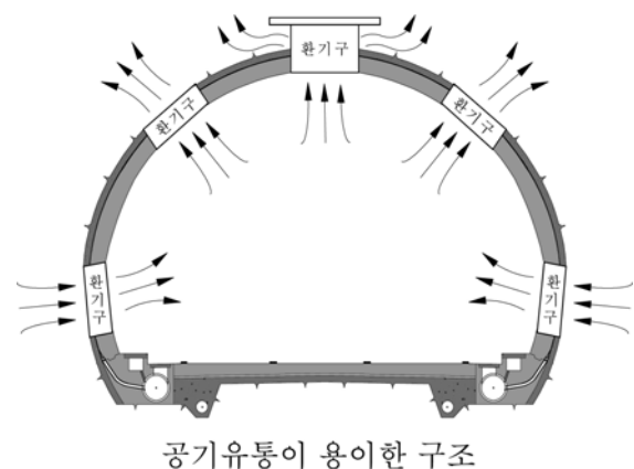
그림 6-42 환기와 매연을 고려한 구조
