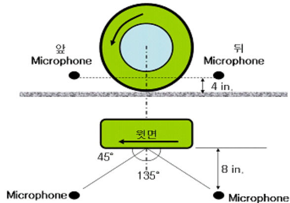
그림 4-30 근접 소음 측정법 마이크론 위치(ISO)
