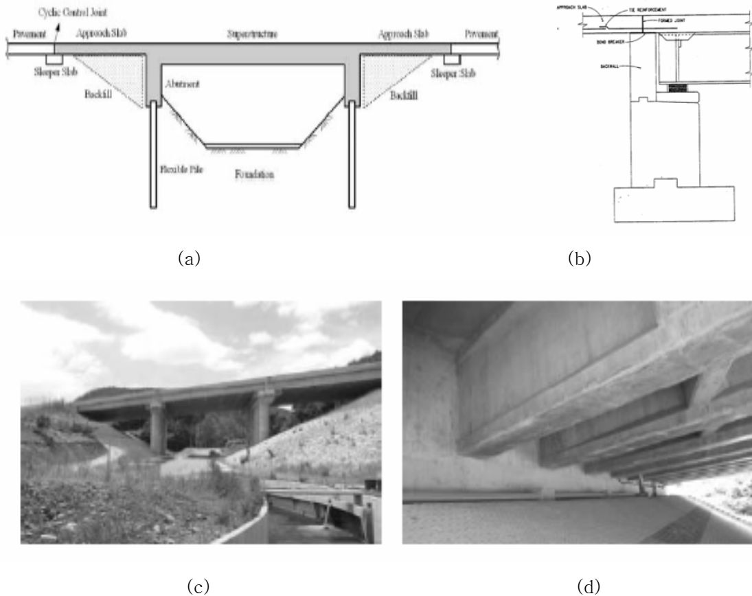
그림 6-17 일체식교대 교량 : (a) 일체식교대 교량의 개념도; (b) 교대부분; (c) 평촌1교 전경; (d) 평촌1교 교대부분
