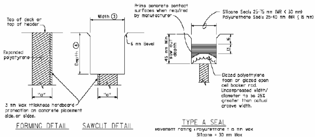
그림 6-5 Caltran의 Type A Joint 상세도
