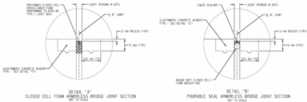
그림 6-7 Armorless joint 시스템-2
