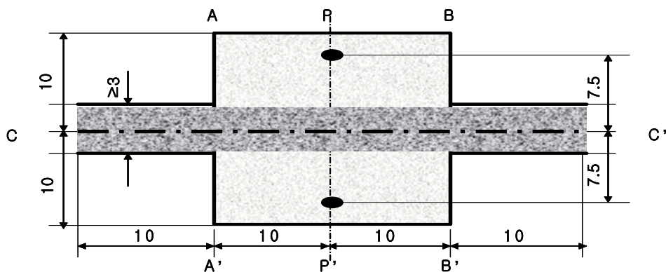
그림 4-26 가속주행소음 시험장(한국, 일본, 유럽)(ISO 362 Working Draft, 2001)
