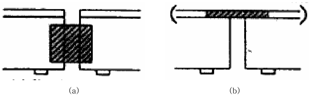
그림 6-19 연결형 무조인트 방식; (a) 휨 모멘트 전달방식, (b) 휨 모멘트 비전달방식
