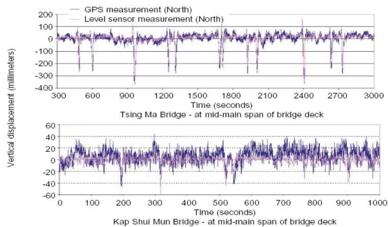
그림 7-11 Level Sensor와 GPS 측정결과의 비교
