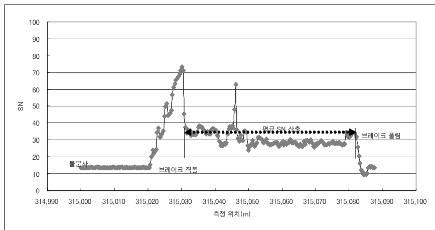
그림 4-44 미끄럼저항 측정 방식
