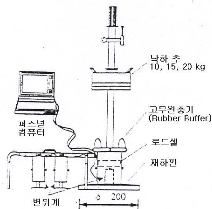
그림 4-15 LFWD의 개략도
