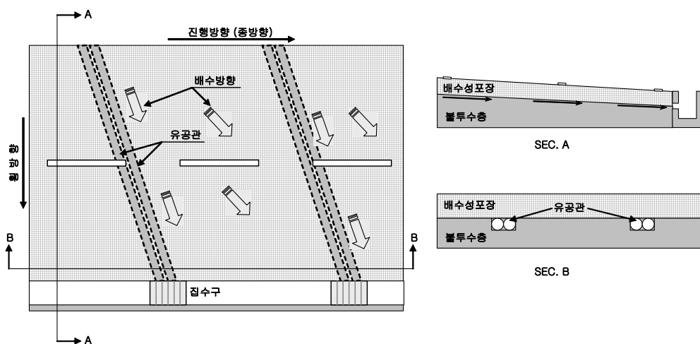
그림 5-16 배수성포장 하부 유공관 매설 (종단경사가 큰 경우)
