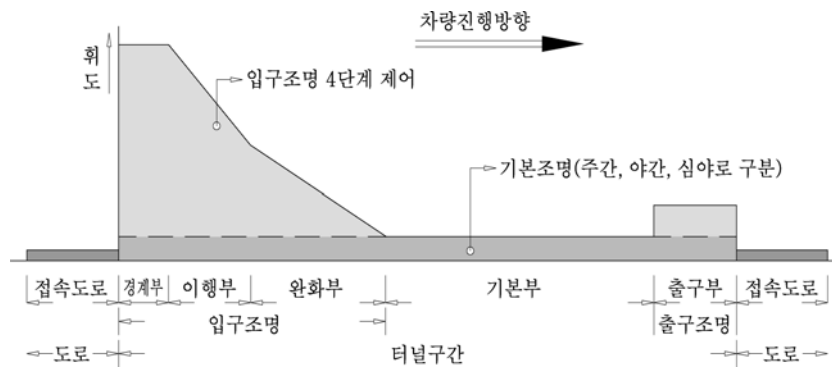
그림 6-36 터널의 노면휘도 분포
