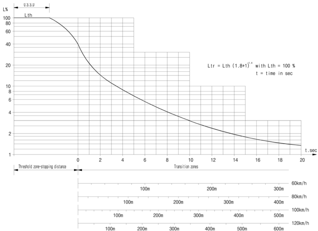
그림 6-46 입구부 조명 휘도 곡선
