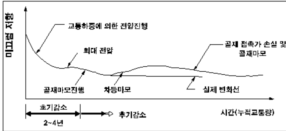
그림 4-43 시간경과에 따른 노면 미끄럼 저항 변화
