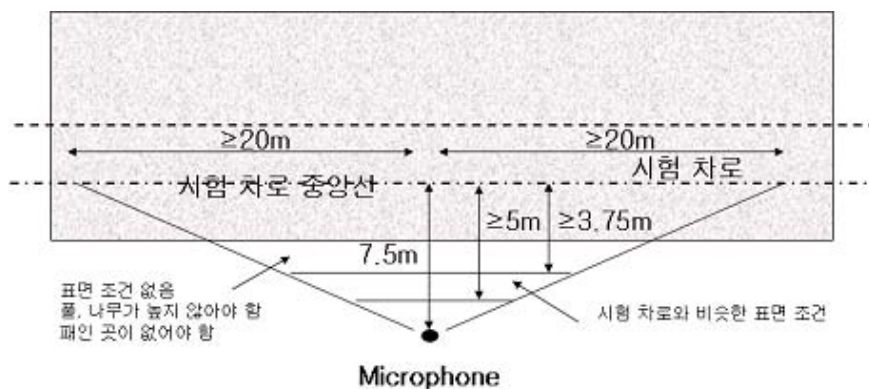
그림 4-23 SPB 소음 측정 조건-2 (ISO 11819-1, 1997)
