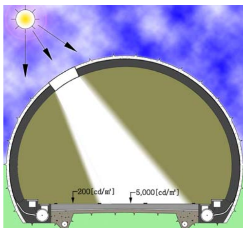
그림 6-41 터널내 직사광에 의한 휘도의 분포
