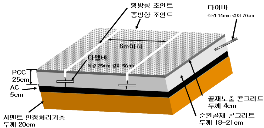
그림 4-8 오스트리아의 이중포설 단면
