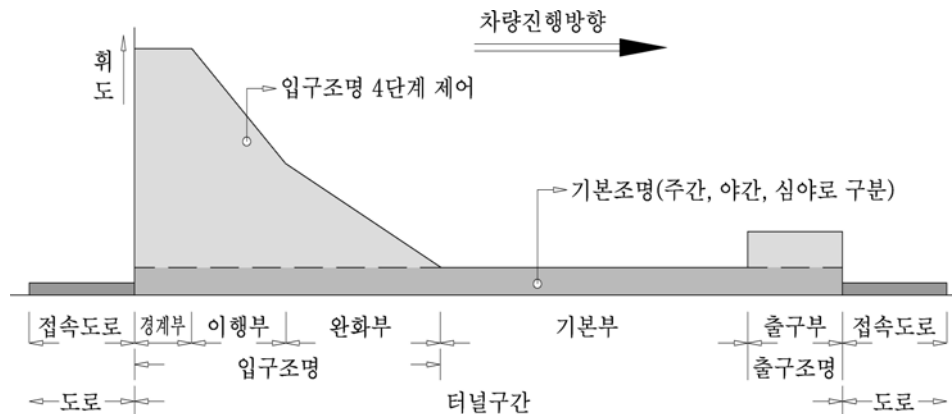
그림 6-44 터널의 노면회도 분포
