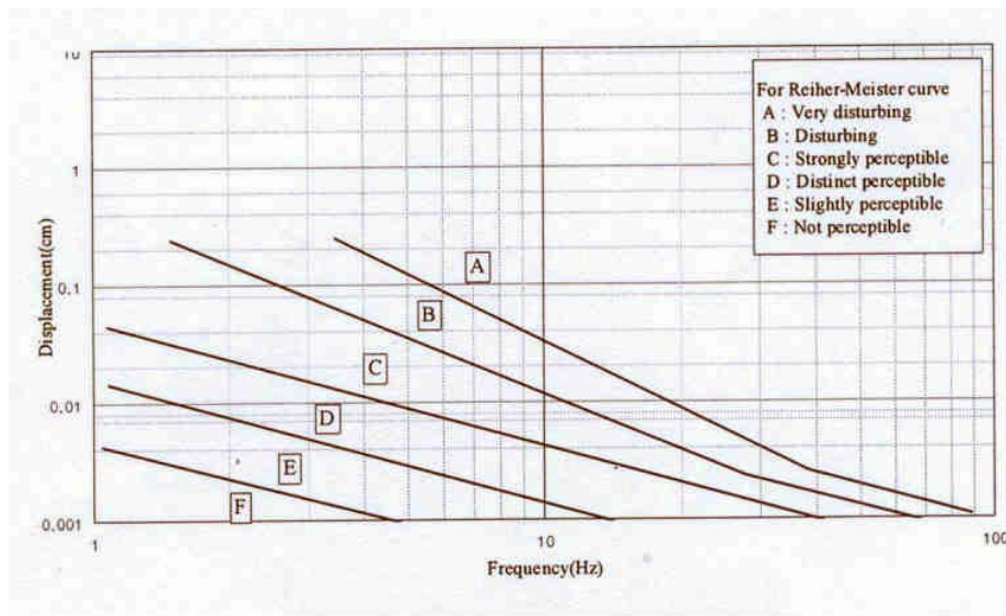
그림 6-10 Reiher-Meister 사용성 허용곡선
