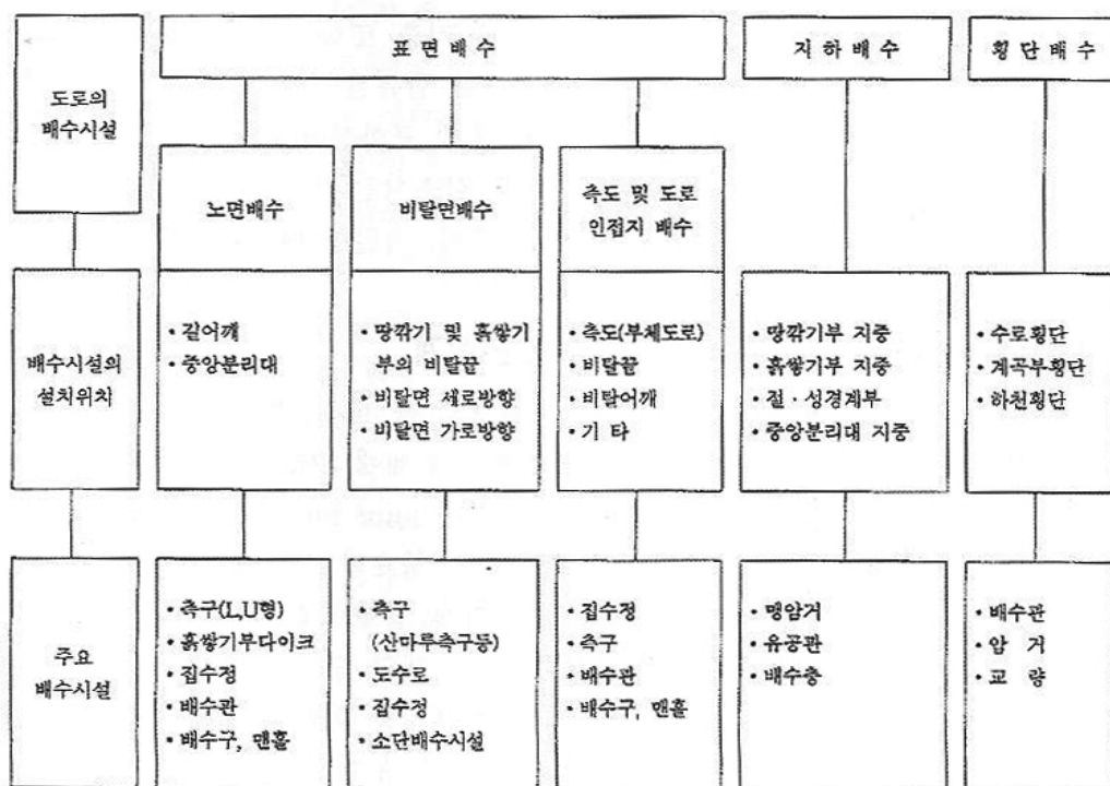
그림 5-12 도로의 배수시설 구분 (도로설계편람, 2000)
