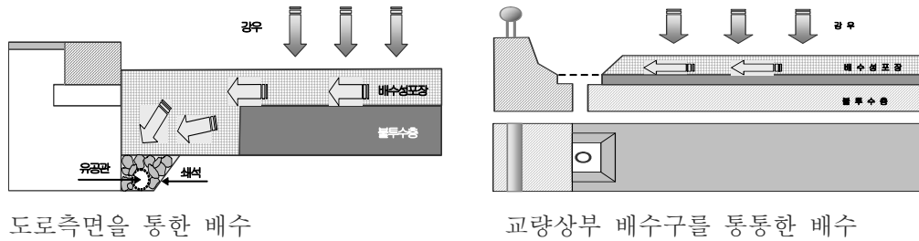
그림 5-15 각 포장별 우수처리 개념도
