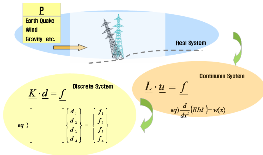
그림 7-9 구조물의 변위 계측에 의한 상태 평가(역해석)
