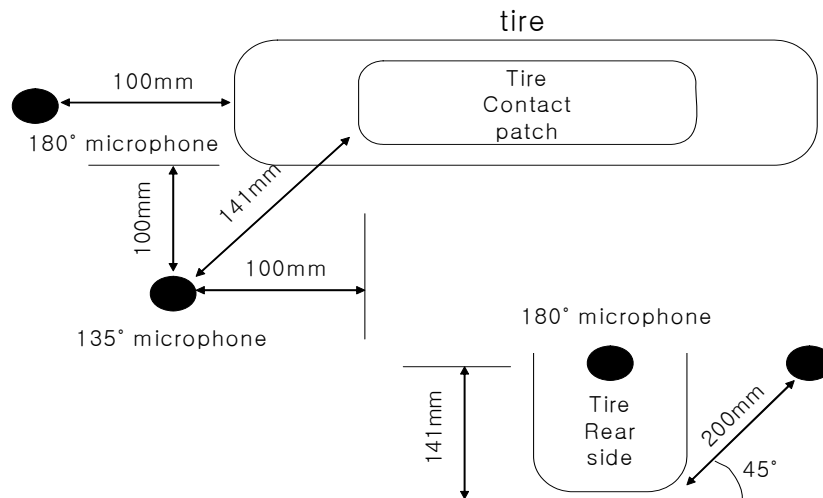
그림 4-32 텍사스 도로국의 근접 소음 측정 마이크론 위치(McNerney, 1998)
