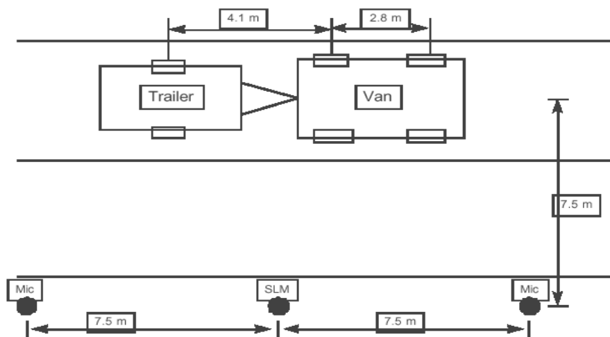
그림 4-31 트레일러를 이용한 소음 측정(McNerney, 1998)
