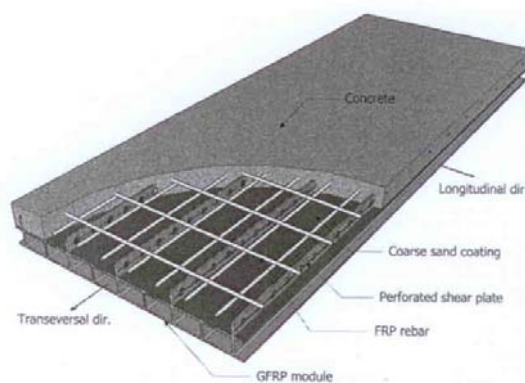
그림 6-14 FRP-콘크리트 합성 바닥판 예9)
