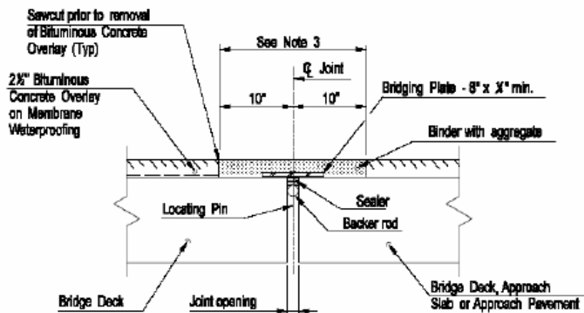
그림 6-8 Asphalt plug joint 시스템
