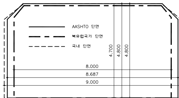
그림 6-28 건축한계 비교
