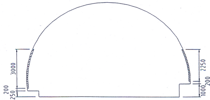
그림 6-31 내장재 세부설치(3m)
