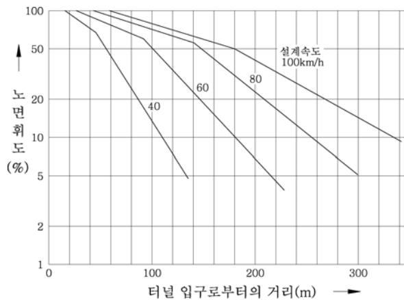
그림 6-37 터널입구의 노면휘도 (KSA 3703)
