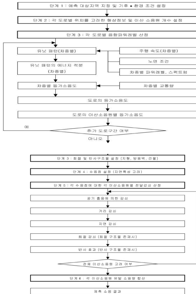
그림 4-40 KHTN-2001 소음 예측 과정
