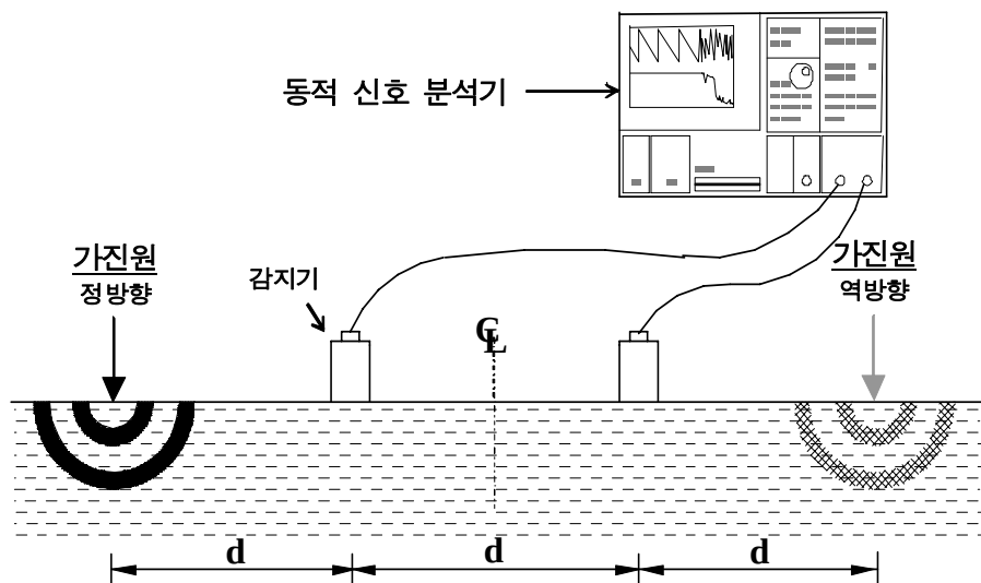
그림 4-16 SASW 시험의 장비 개요도
