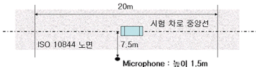
그림 4-25 단독차량 pass-by method(ISO)
