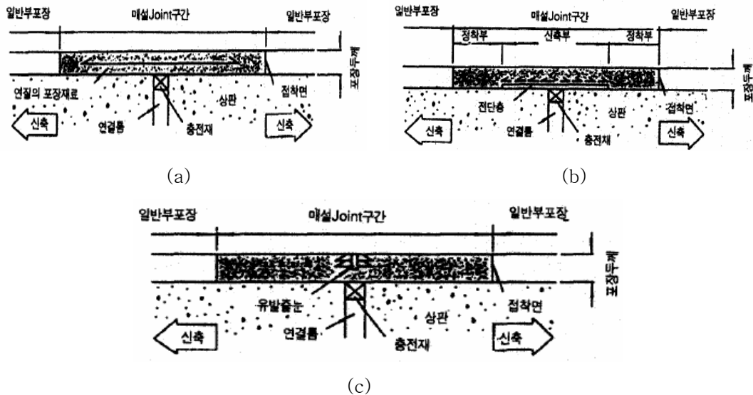
그림 6-18 매설형 무조인트 방식의 종류
