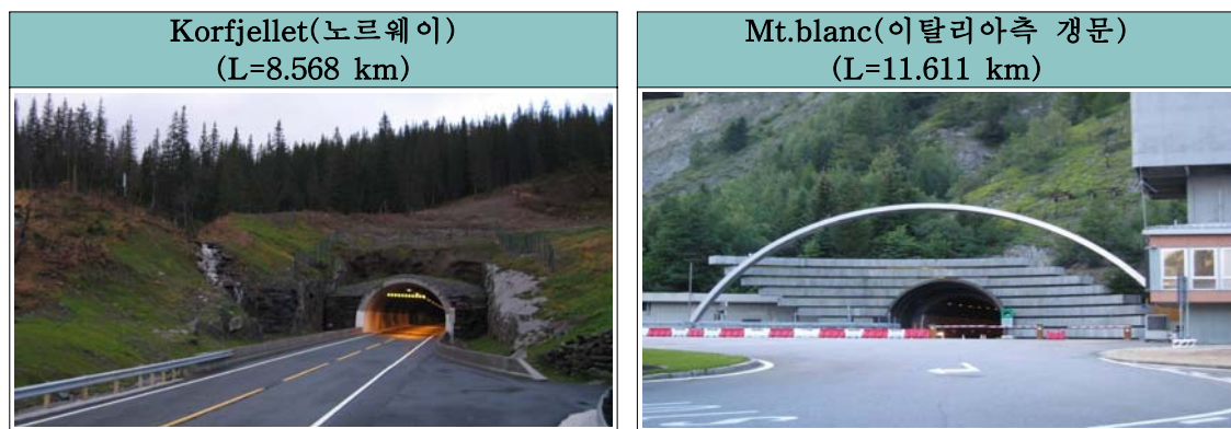
그림 6-26 유럽의 터널갱문 적용사례
