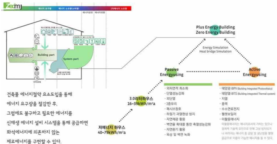
[그림1.7] 제로에너지 건축물 (출처: 이명주(주)제드애펬이 건축사사무소)
