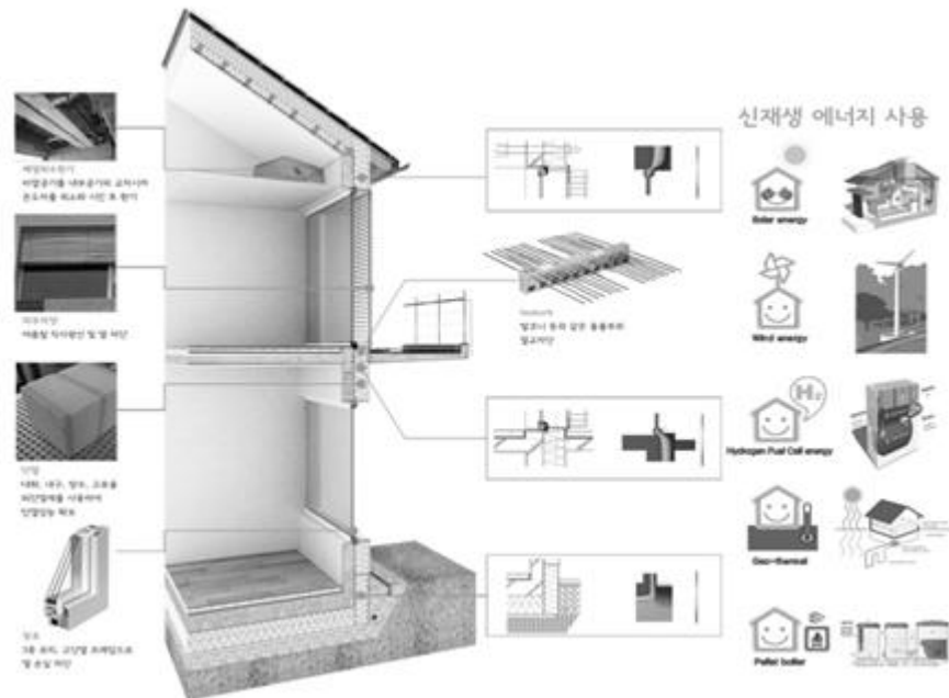
[그림2.4] 건축물 단계별 프로세스 및 제로에너지주택적용기술 (출처: (주)제드엠케이 건축사사무소)
