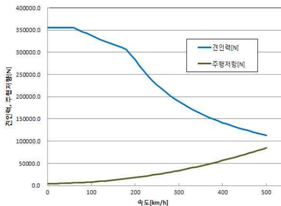
[4M+2MC* 견인력 선도와 주행저항]
