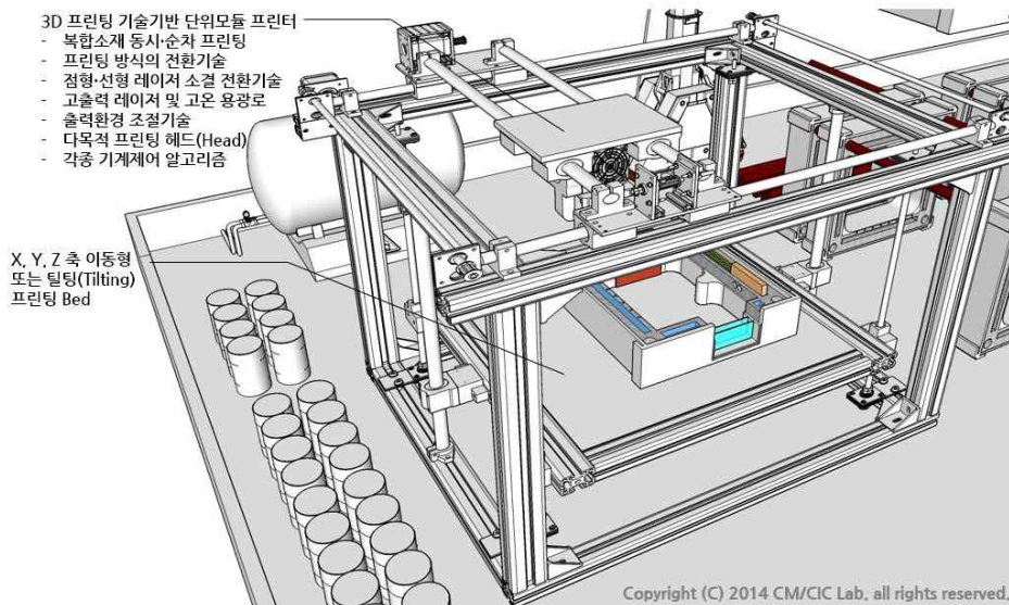
[그림 58] 모듈 프린팅 Zone(예시)
