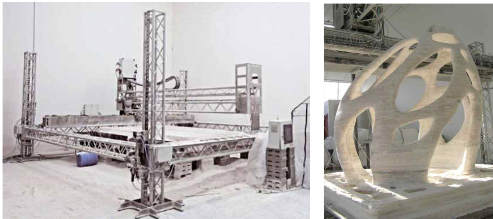
[그림 44] D-shape의 3 D프린터와 제작 결과물
