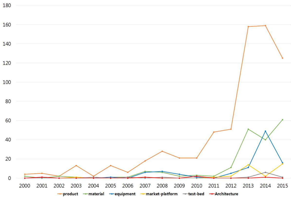
[그림 55] 연도별 국외 3D 프린터 관련 논문 세부 분야 동향
