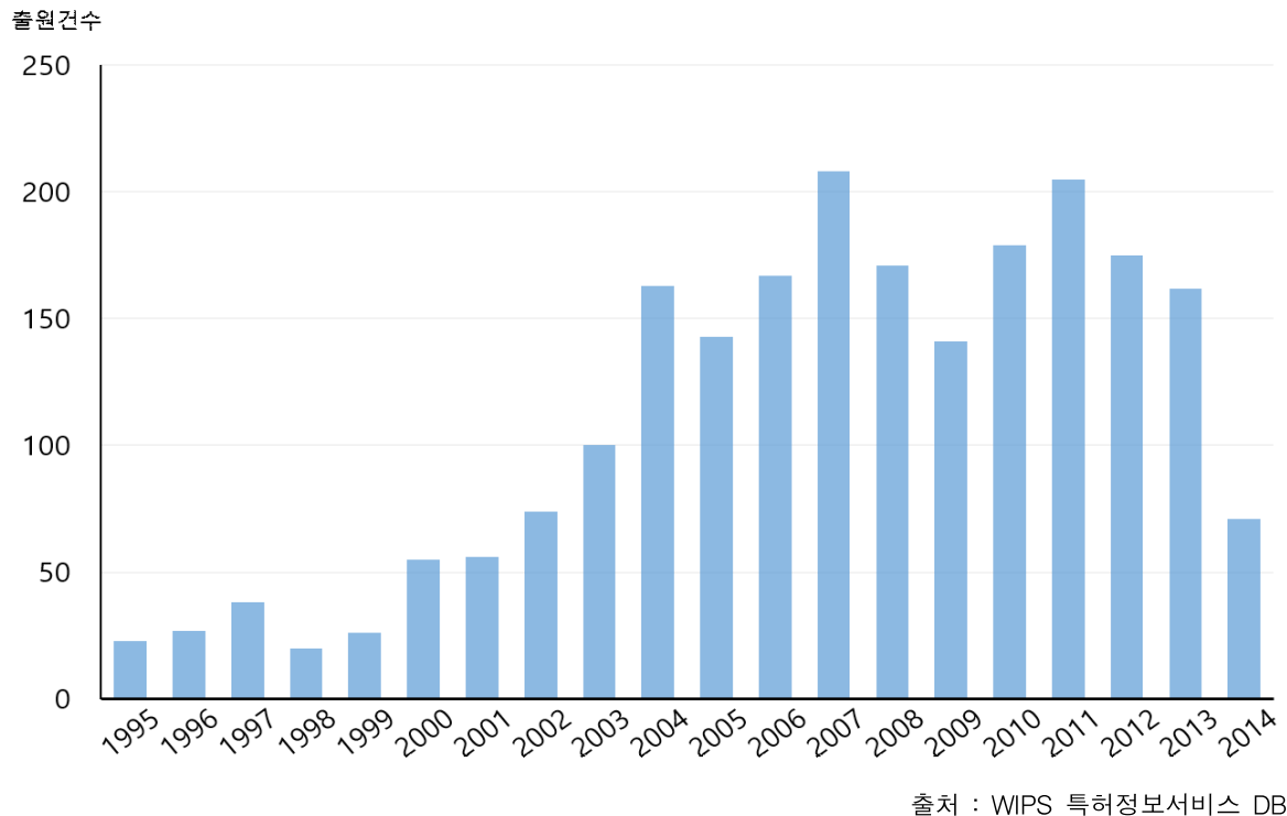
[그림 14] 연도별 미국 3D 프린팅 관련 특허 출원 건수
