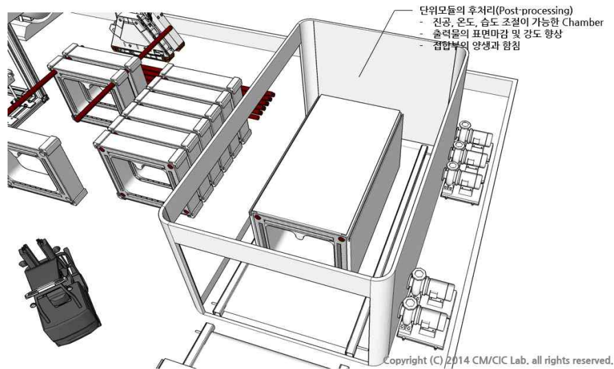
[그림 60] 모듈 양생 및 함침 Chamber Zone(예시)
