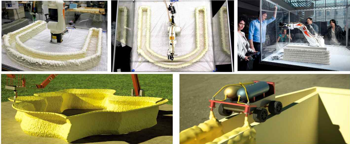
폴리우레탄을 재료로 3D 프린팅 하여 비정형 구조체 생산에 필요한 비정형 거푸집 제작
