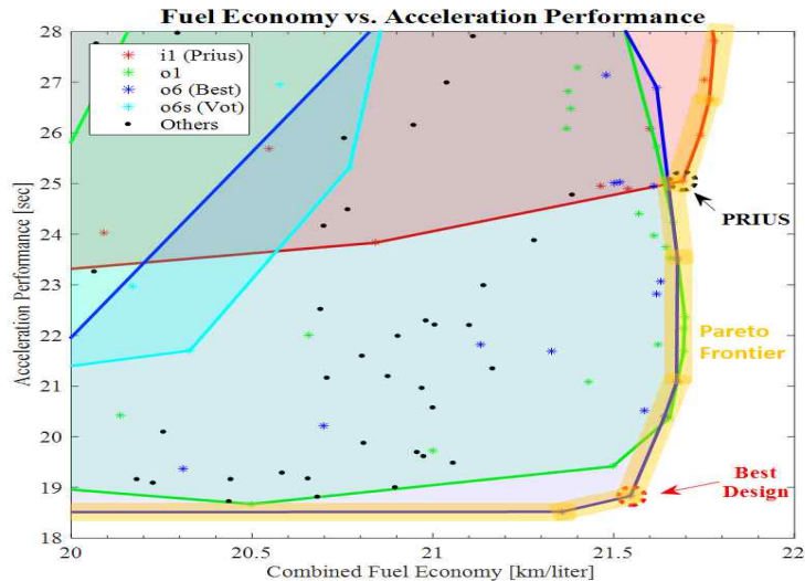
<그림 59> 하이브리드 차량 파워트레인 잠재 성능 평가맵 사례
