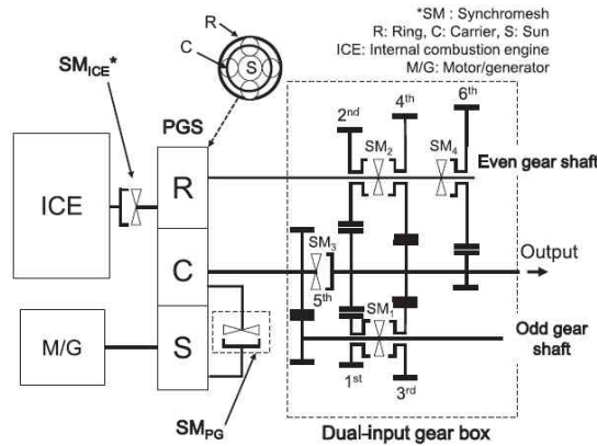
<그림 12> CGST의 파워트레인 구조
