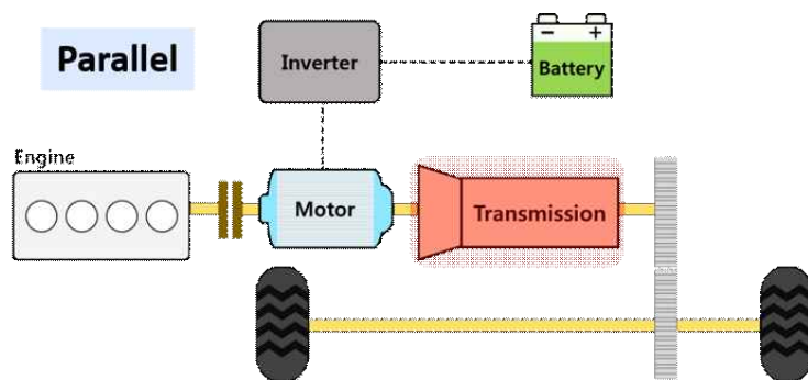
<그림 10> 병렬형 하이브리드 차량의 구조
