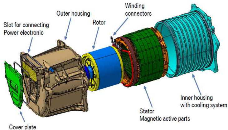
<그림 32> BMW社の i8모델에 적용된 영구자석형 구동 모터
