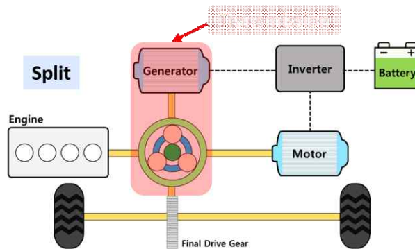
<그림 27> 동력분기형 하이브리드 시스템
