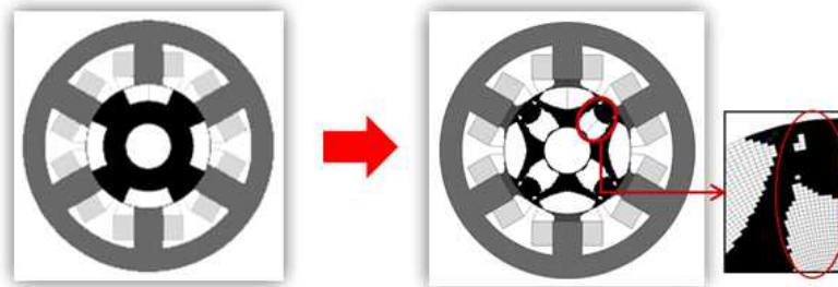
<그림 19> 위상최적설계의 적용을 통한 전기모터의 경량화 연구 사례
