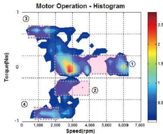
<그림 17> 하이브리드 차량용 모터의 주 사용영역
