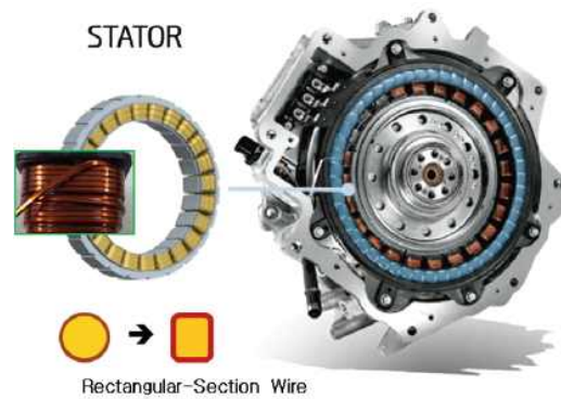
<그림 18> 다중 슬롯·집중권·사각권선을 적용한 구동 모터의 예
