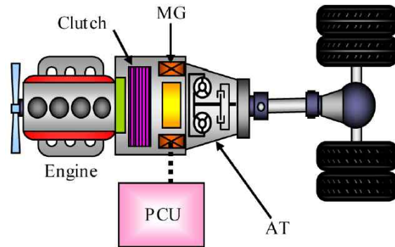
<그림 30> Hino 社 하이브리드 전기 트럭의 병렬형 파워트레인
