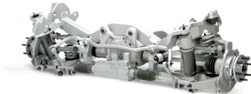
<그림 36> I-Ride 社の 서스펜션 모듈
