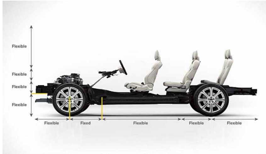
<그림 35> 볼보 社の SPA 모듈화 플랫폼
