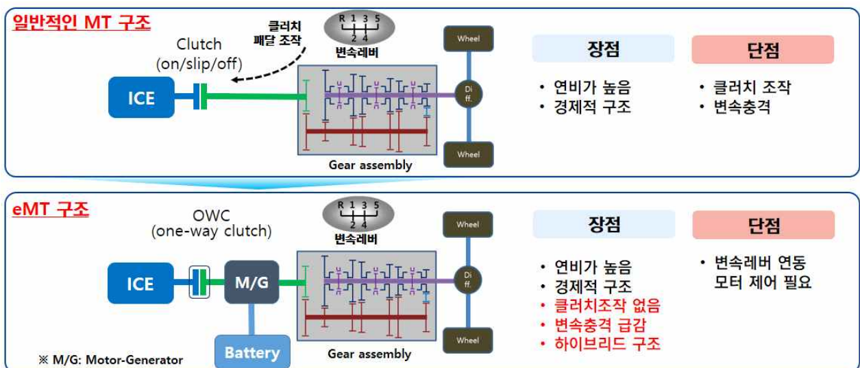
<그림 13> 수동변속기(MT)와 eMT의 파워트레인 구조
