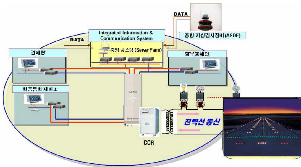
<그림 2-13> 제주국제공항의 개별등화제어시스템 (ILCMS) 구성
