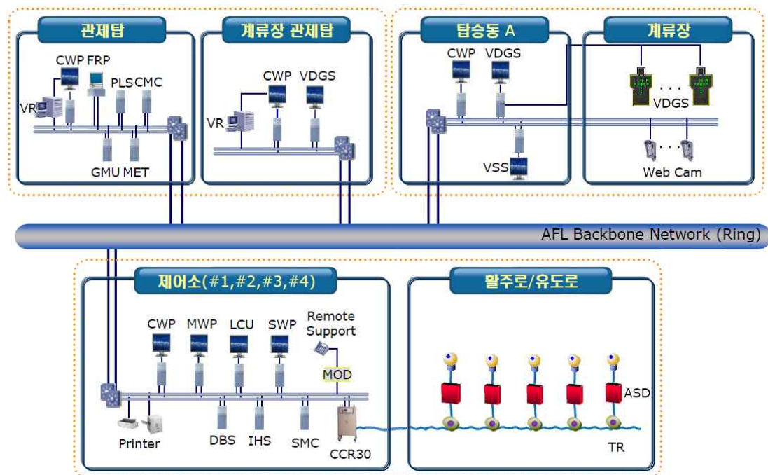
<그림 2-12> 인천국제공항의 개별등화제어시스템 (ILCMS) 구성
